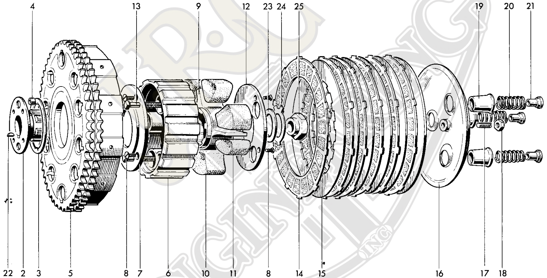
Fig. 9. CLUTCH
