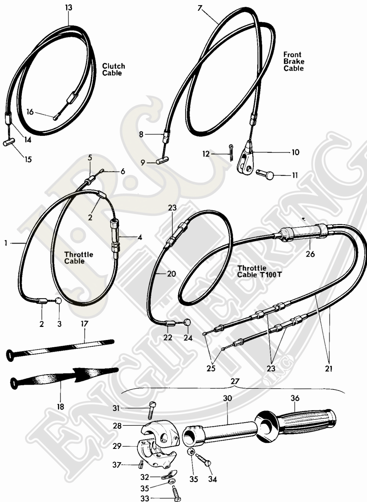
Fig. 28. CONTROL CABLES
