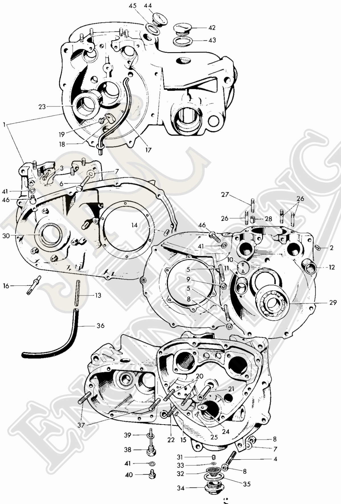
Fig. 2. CRANKCASE
