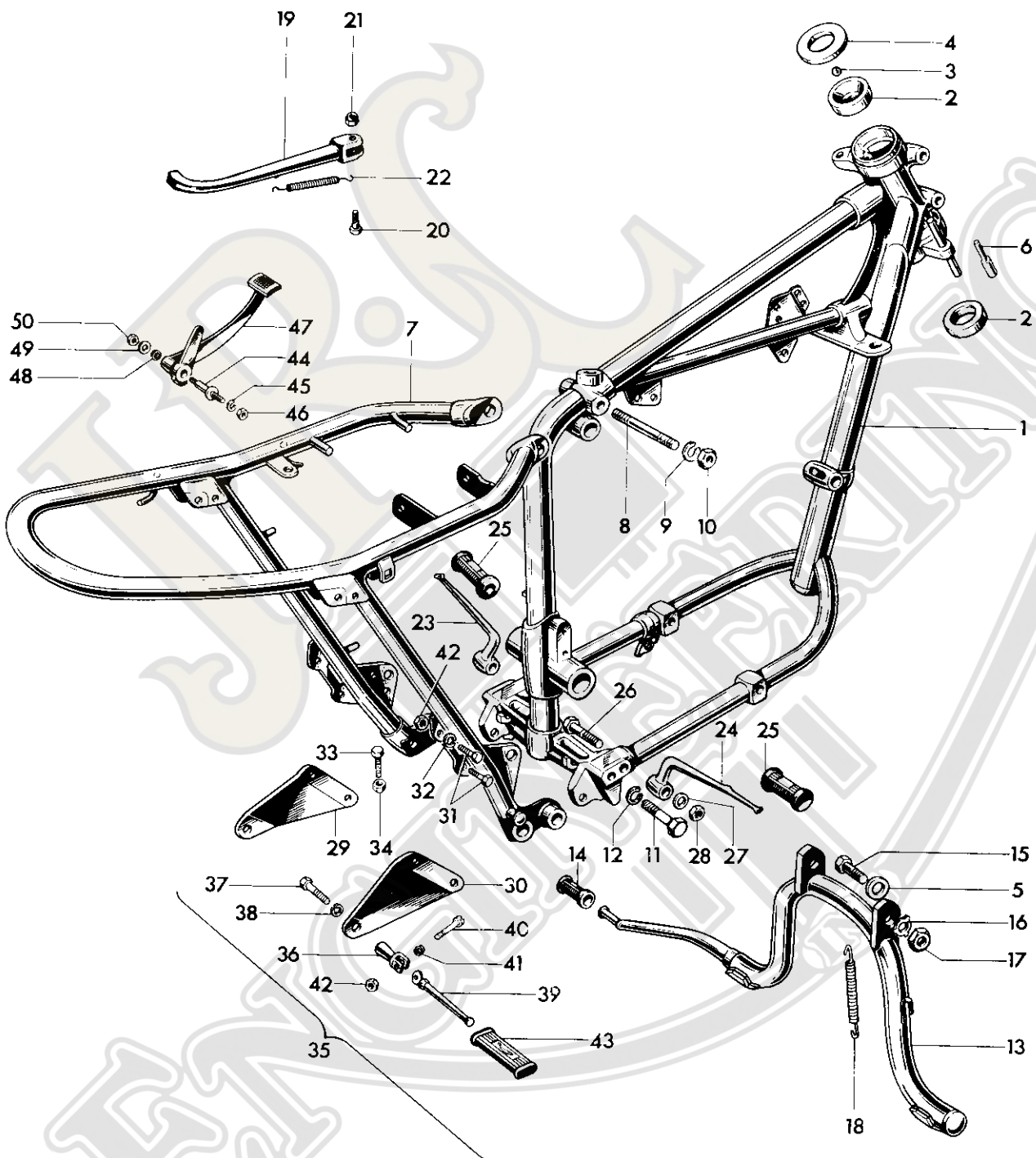
Fig. 15. FRAME
