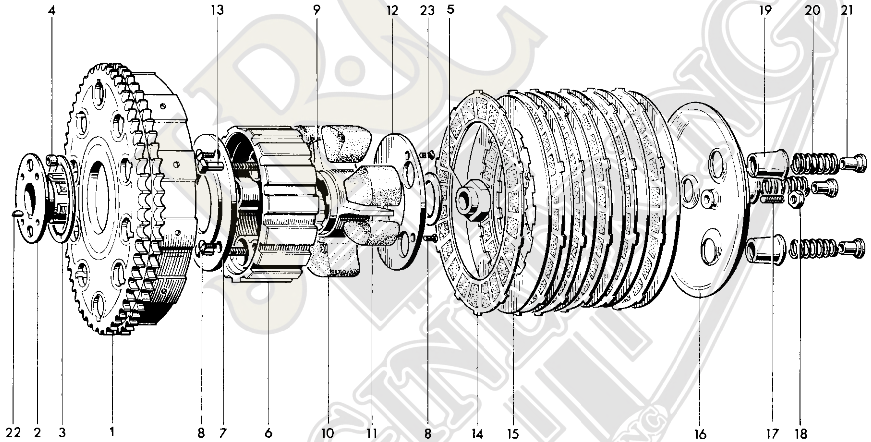
Fig. 11. CLUTCH
