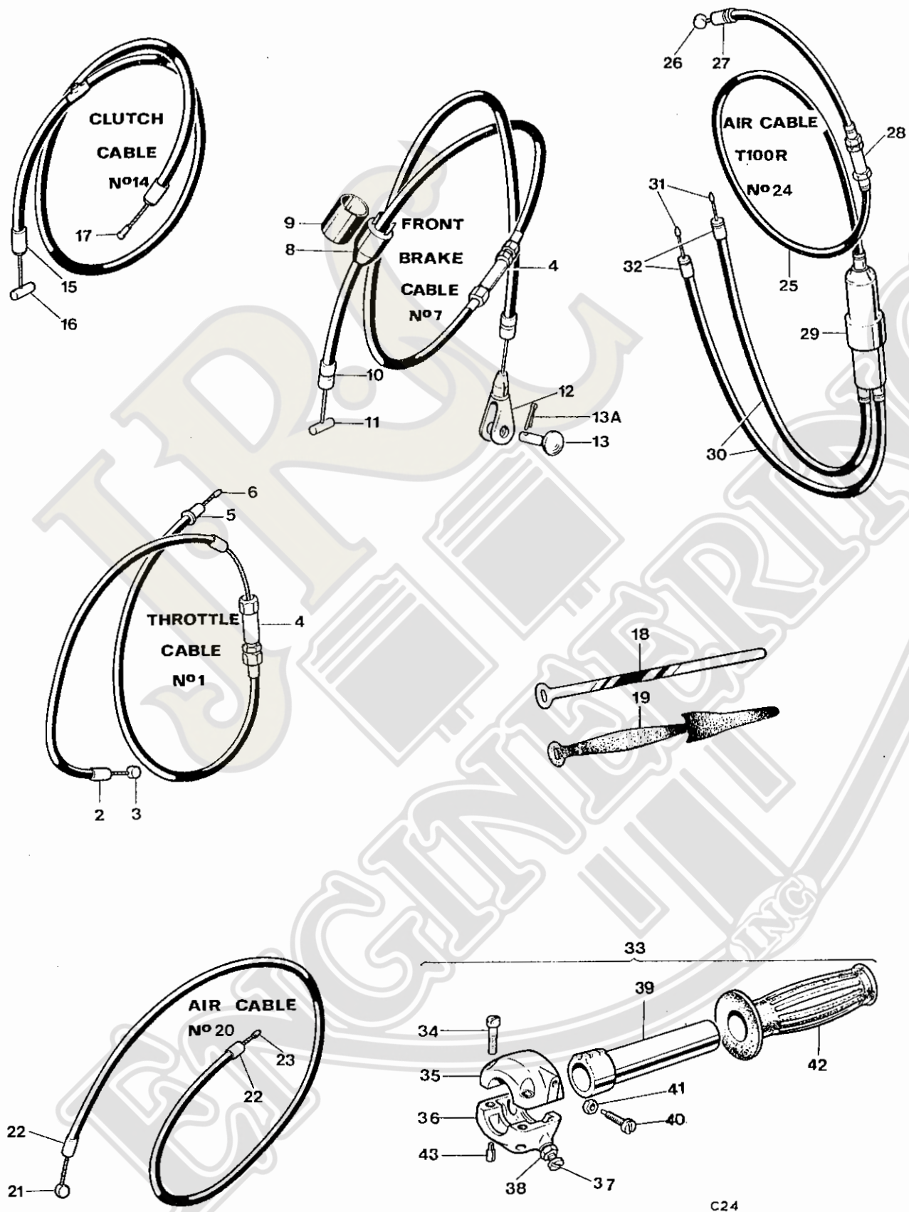
Fig. 29. CONTROL CABLES
