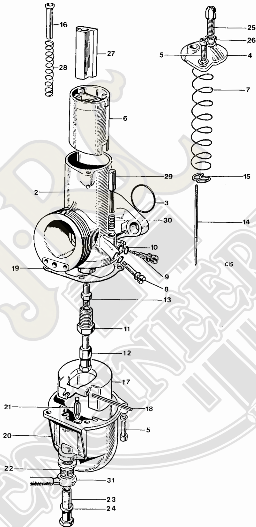
Fig. 31. CARBURETOR T100R
