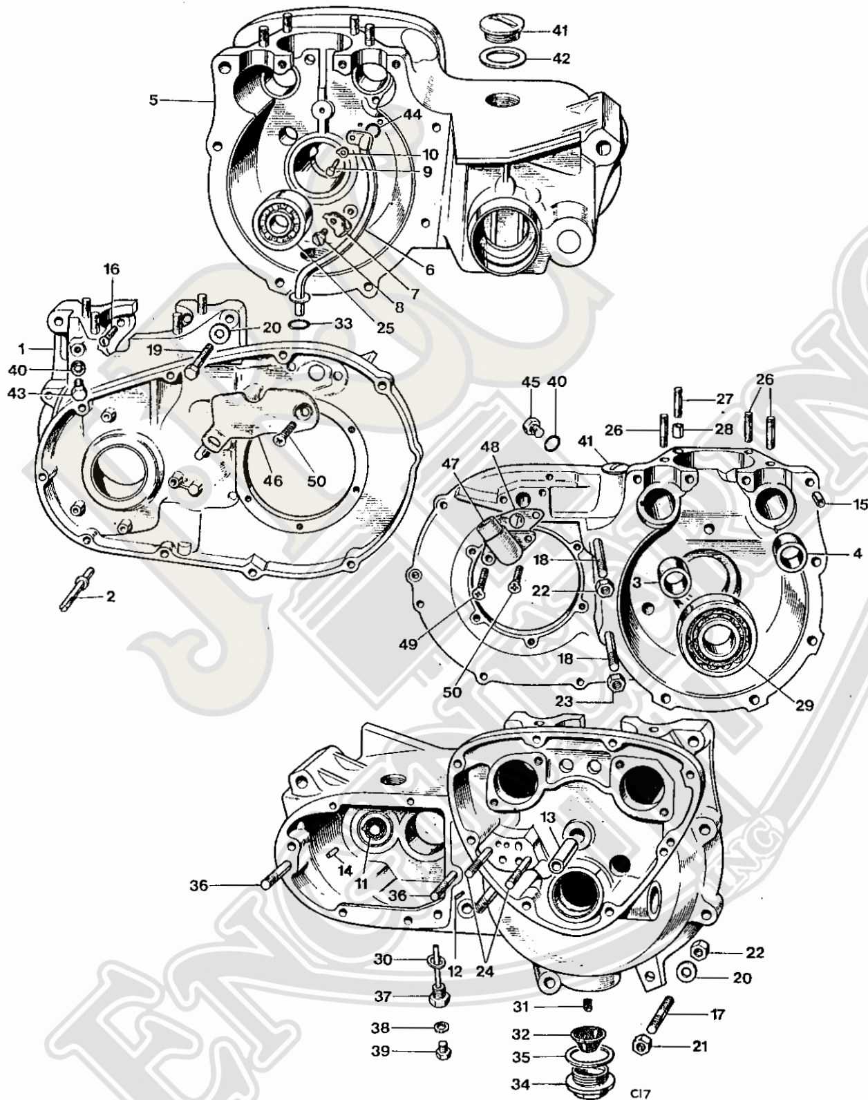
Fig. 2. CRANKCASE
