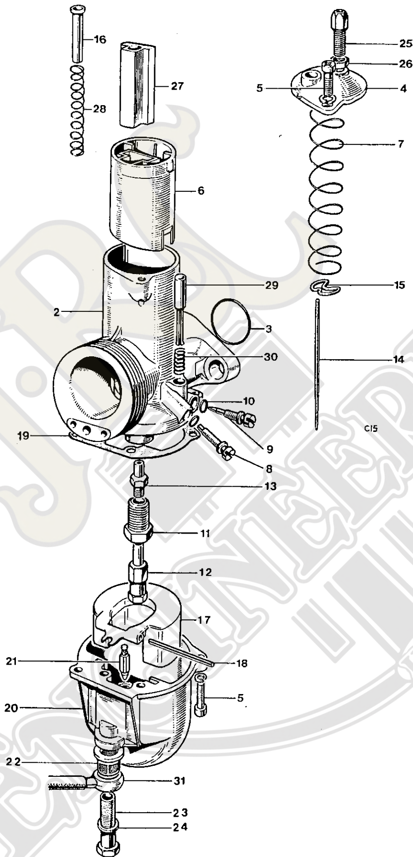
Fig. 30. CARBURETOR T100C
