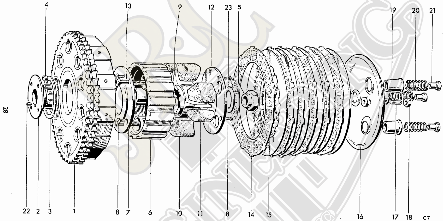
Fig. 11. CLUTCH
