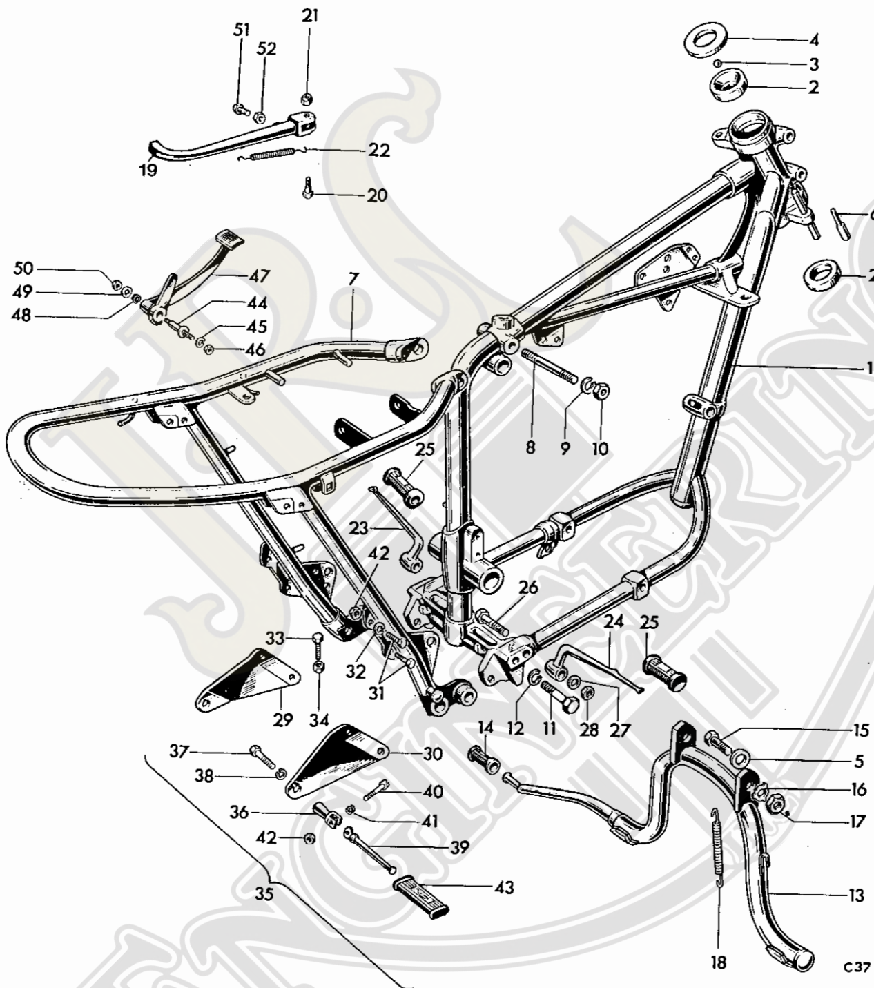
Fig. 15. FRAME
