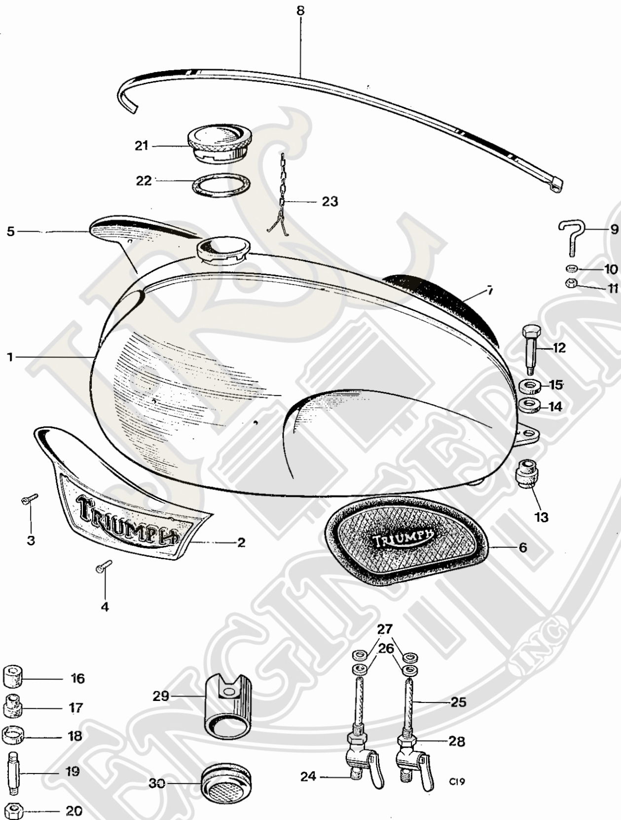
Fig. 25. GAS TANK
