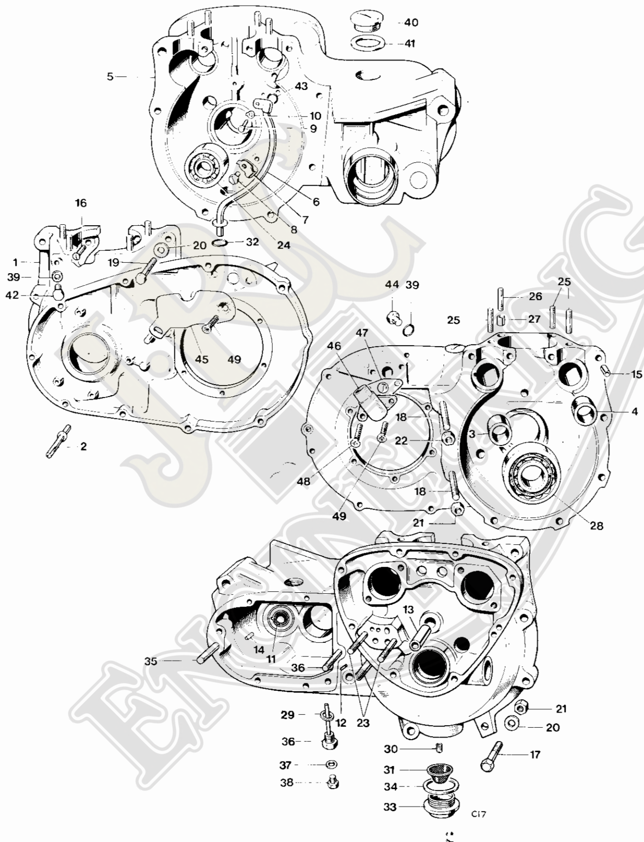
Fig. 2. CRANKCASE
