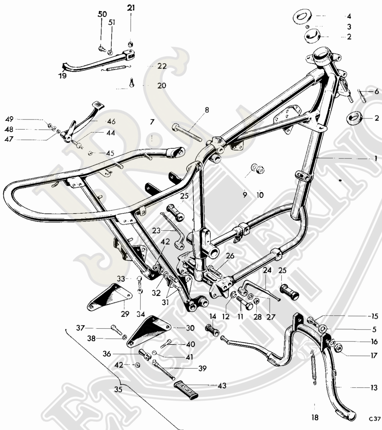
Fig. 18. FRAME
