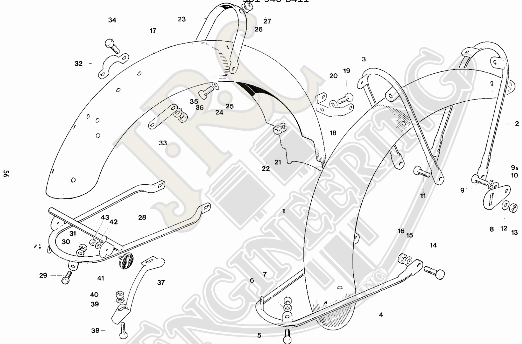
Fig. 24. FENDERS
