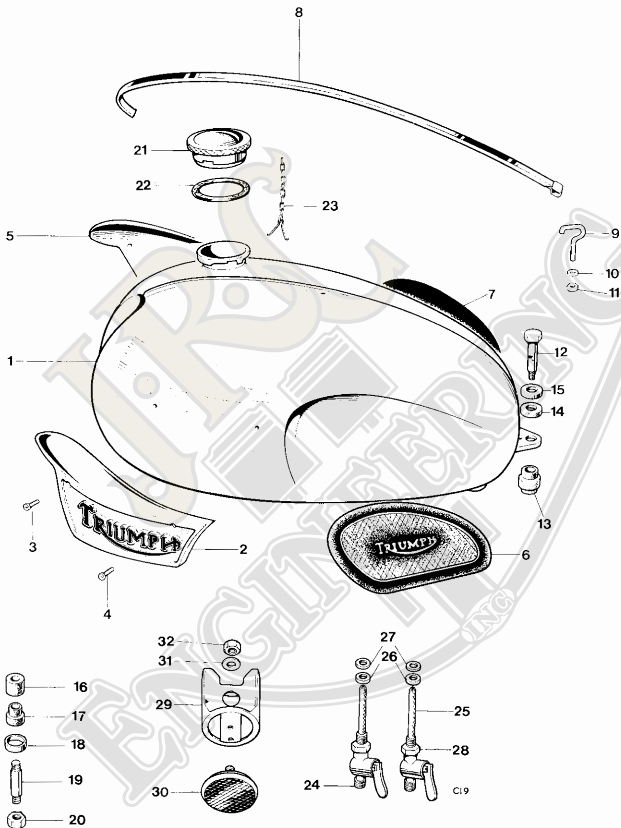
Fig. 27. GAS TANK
