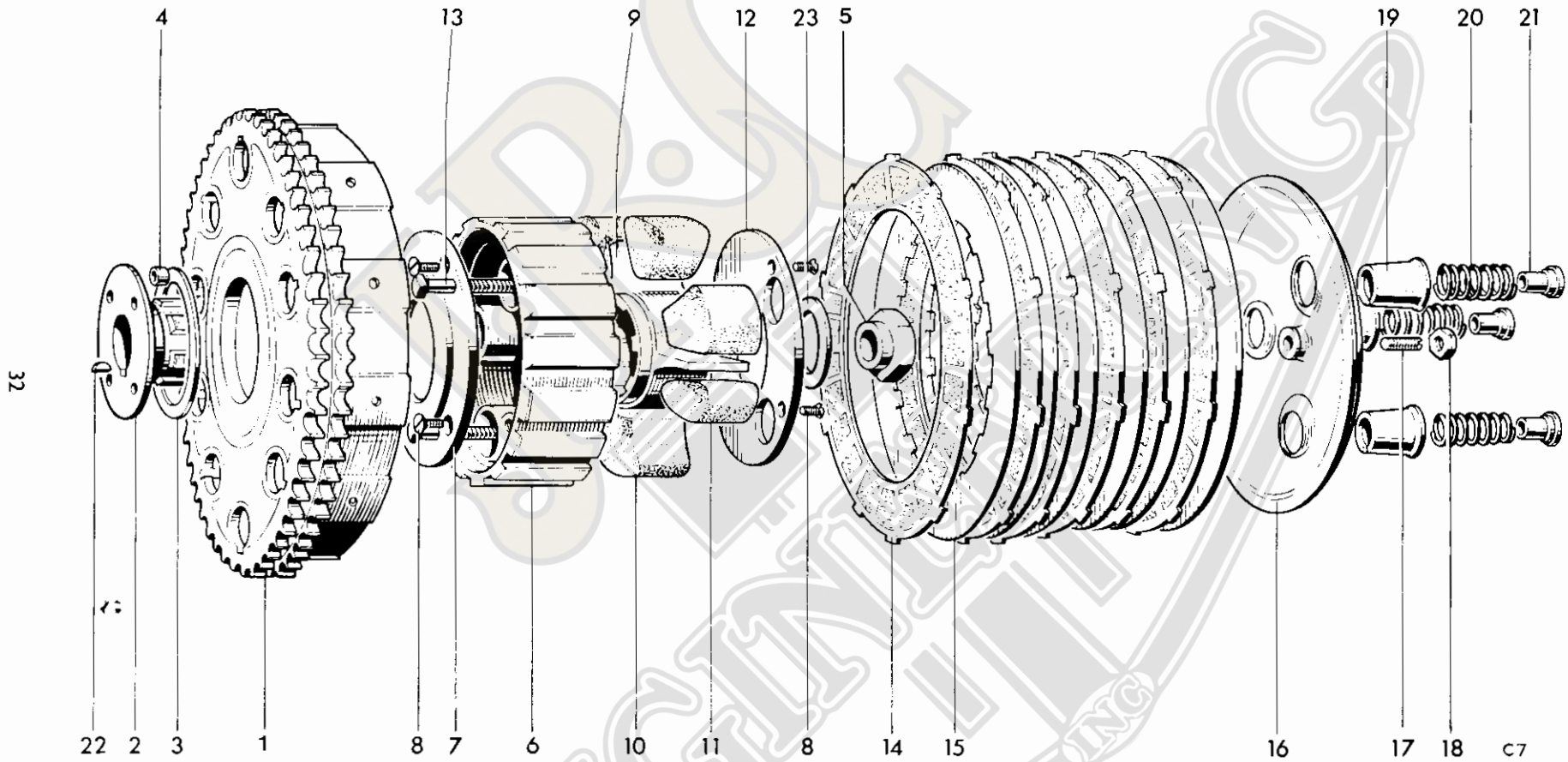
Fig. 13. CLUTCH
