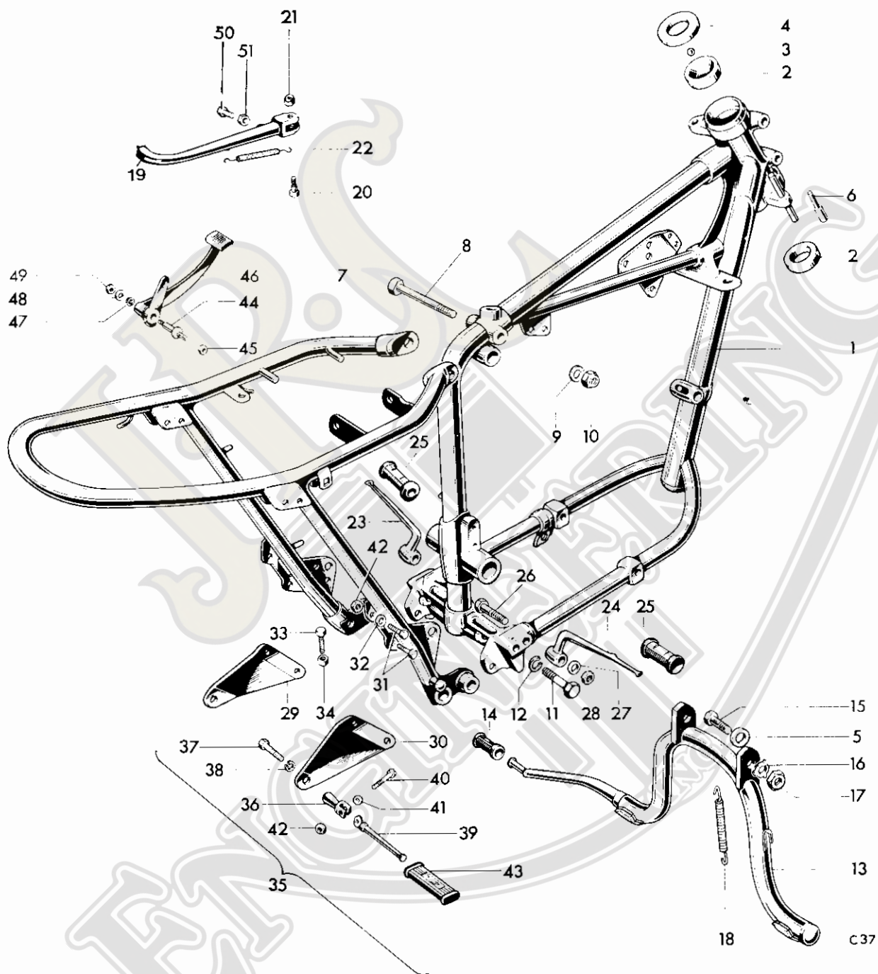
Fig. 14. FRAME
