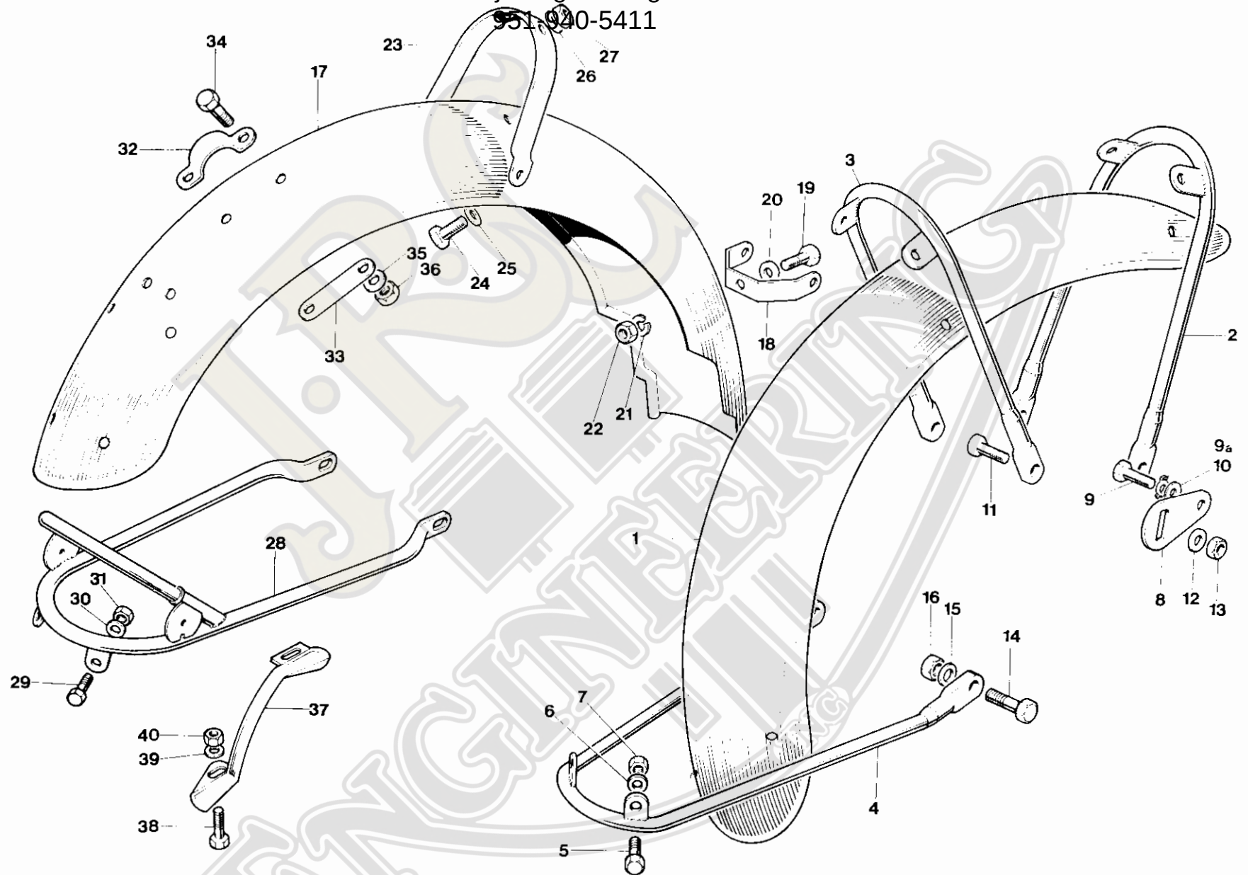
Fig. 19. FENDERS
