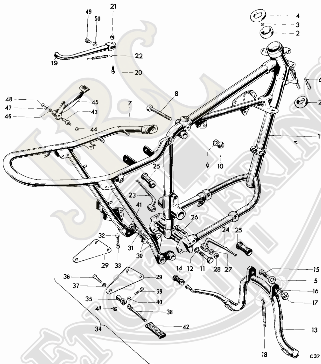
Fig. 14. FRAME
