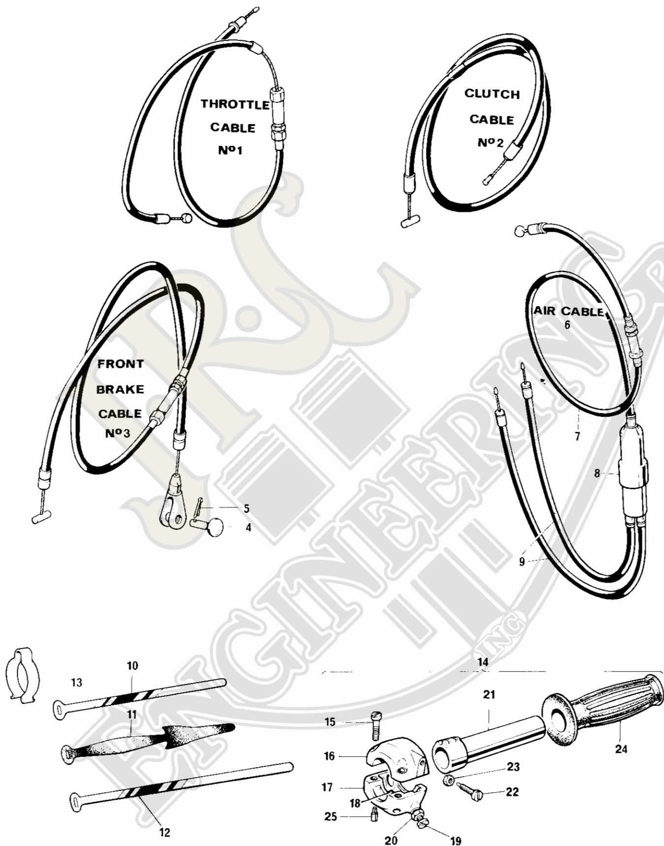
Fig. 26. CONTROL CABLES
