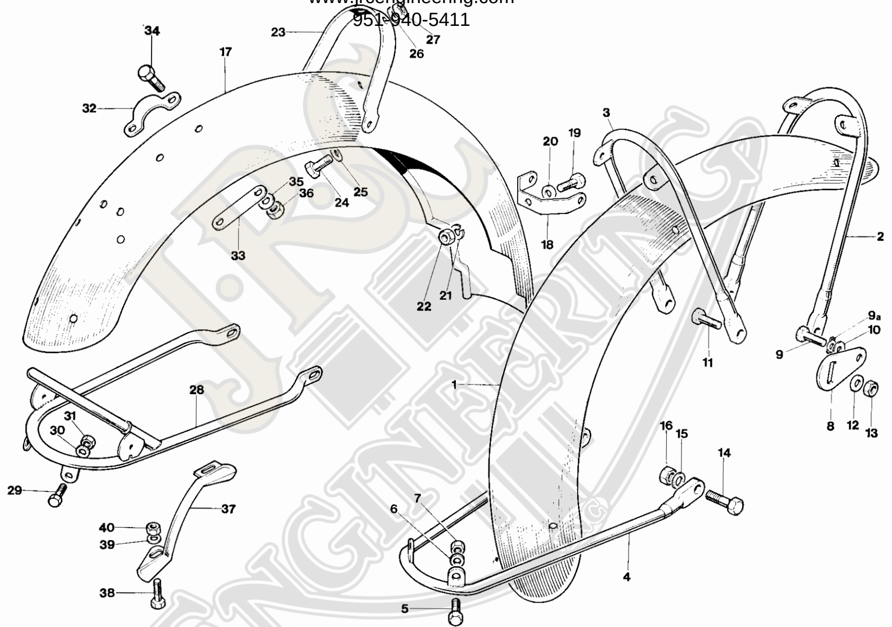
Fig. 19. FENDERS
