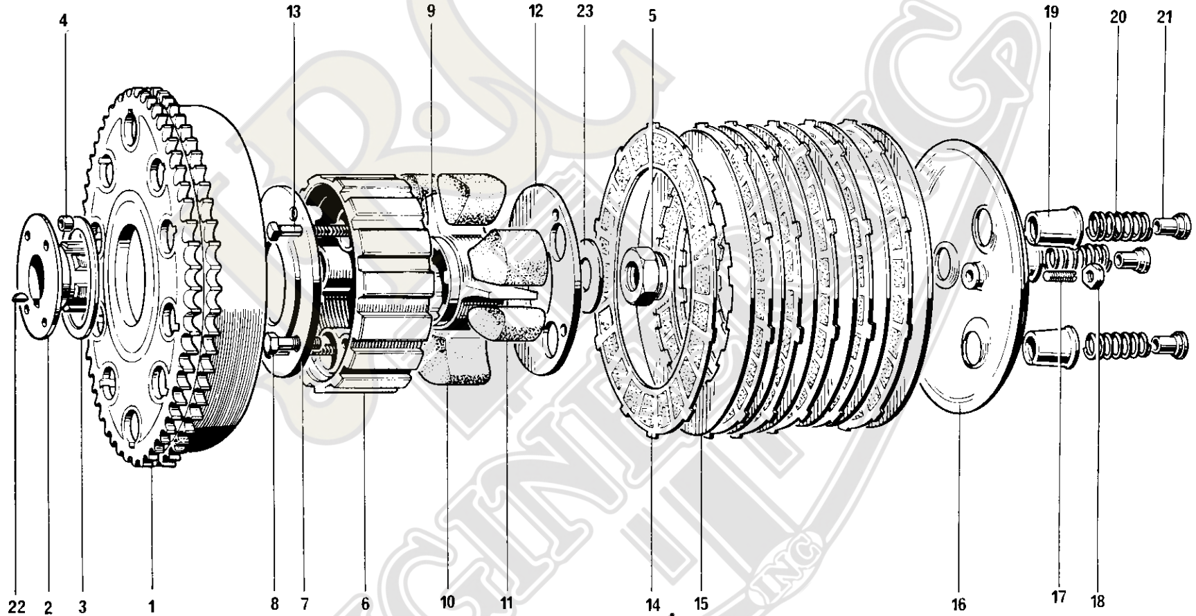
Fig. 10. CLUTCH
