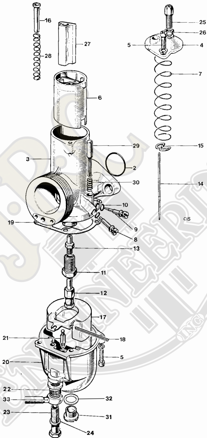
Fig. 5. CARBURETOR
