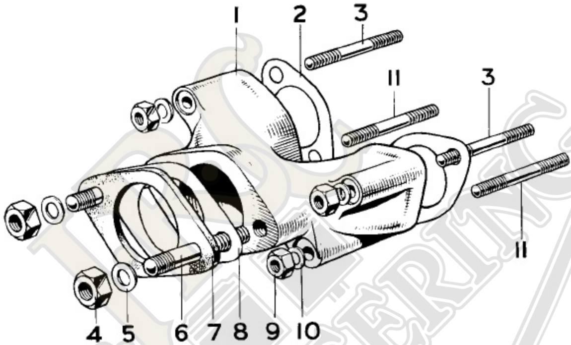
FIG. I INLET MANIFOLD
