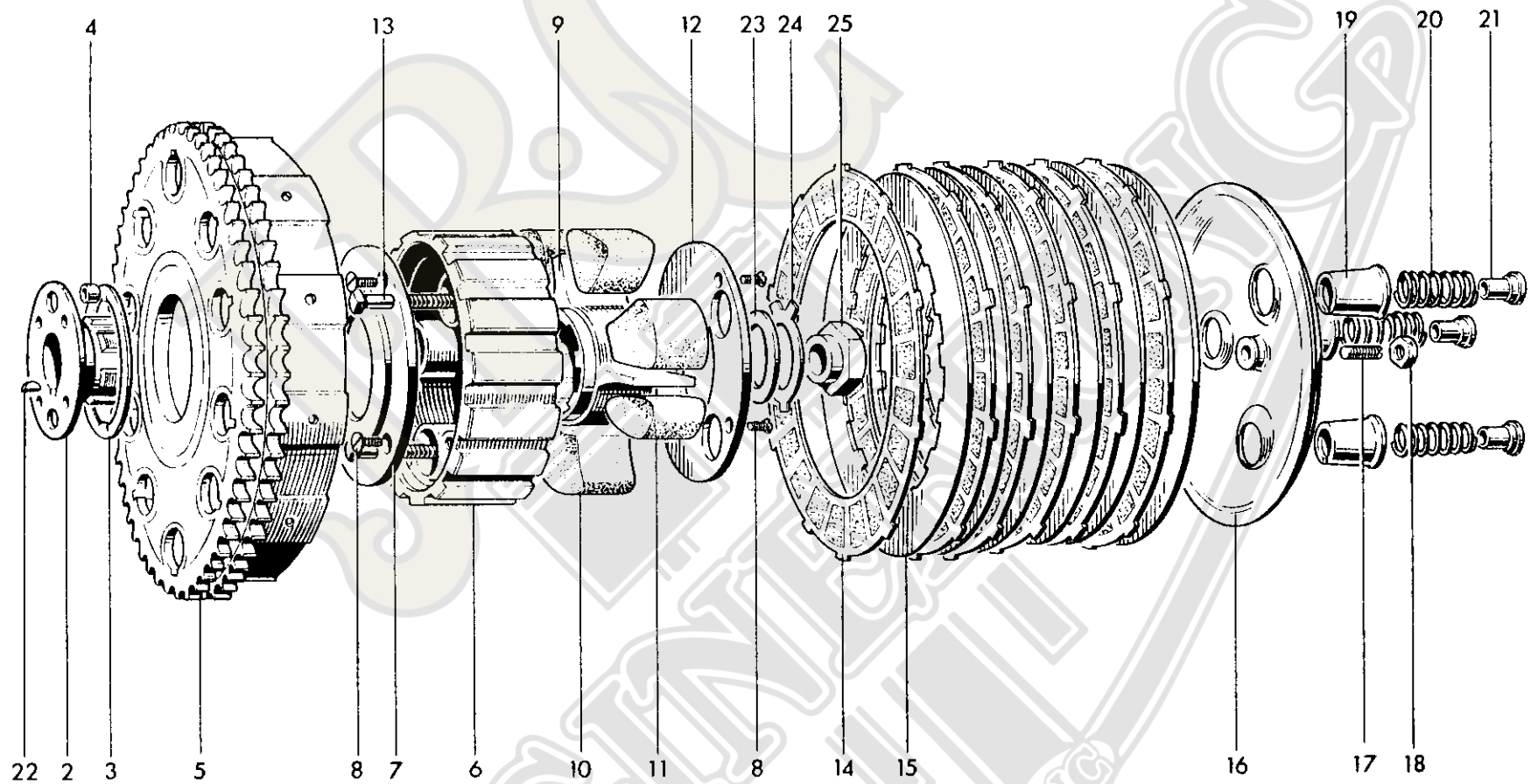
Fig. 10. CLUTCH
