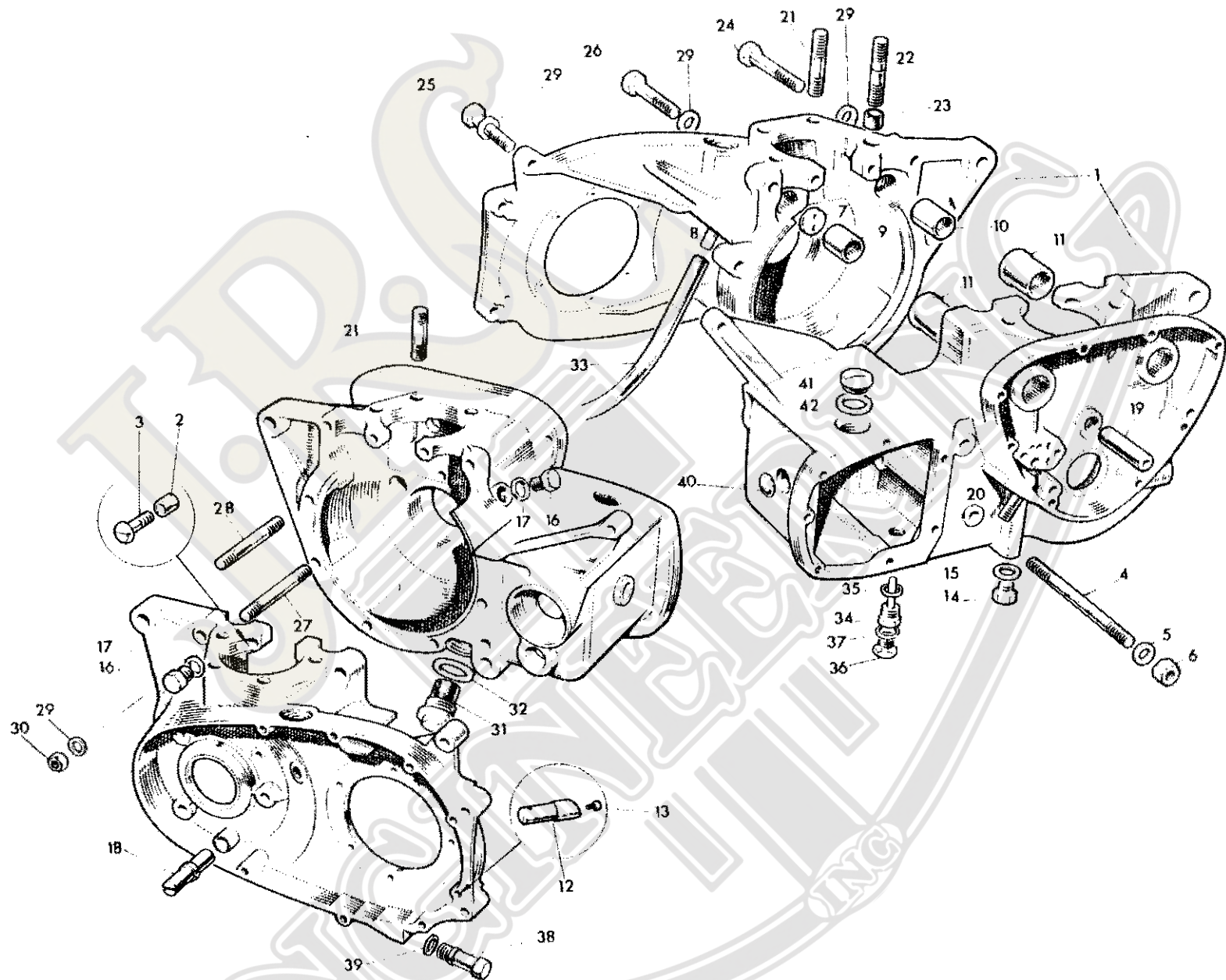
Fig. 2. CRANKCASE
