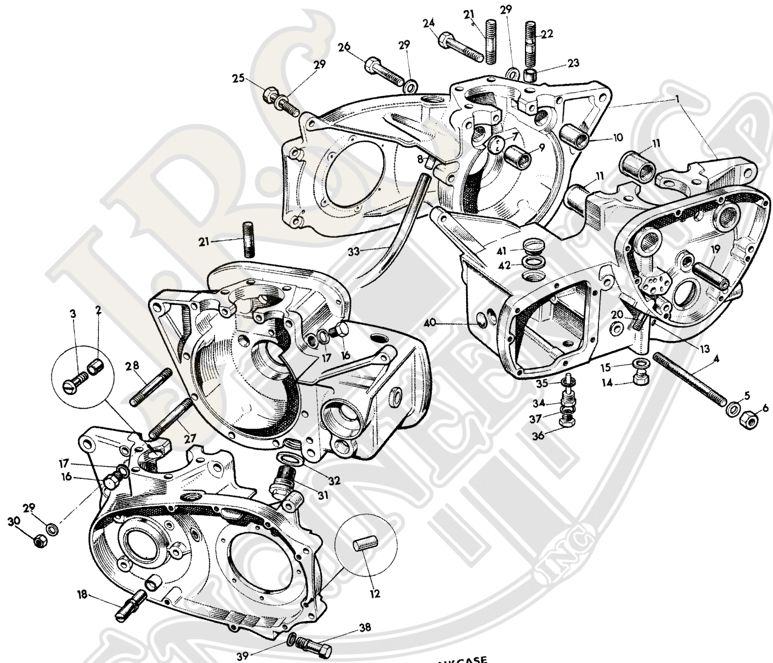
Fig. 2. CRANKCASE
