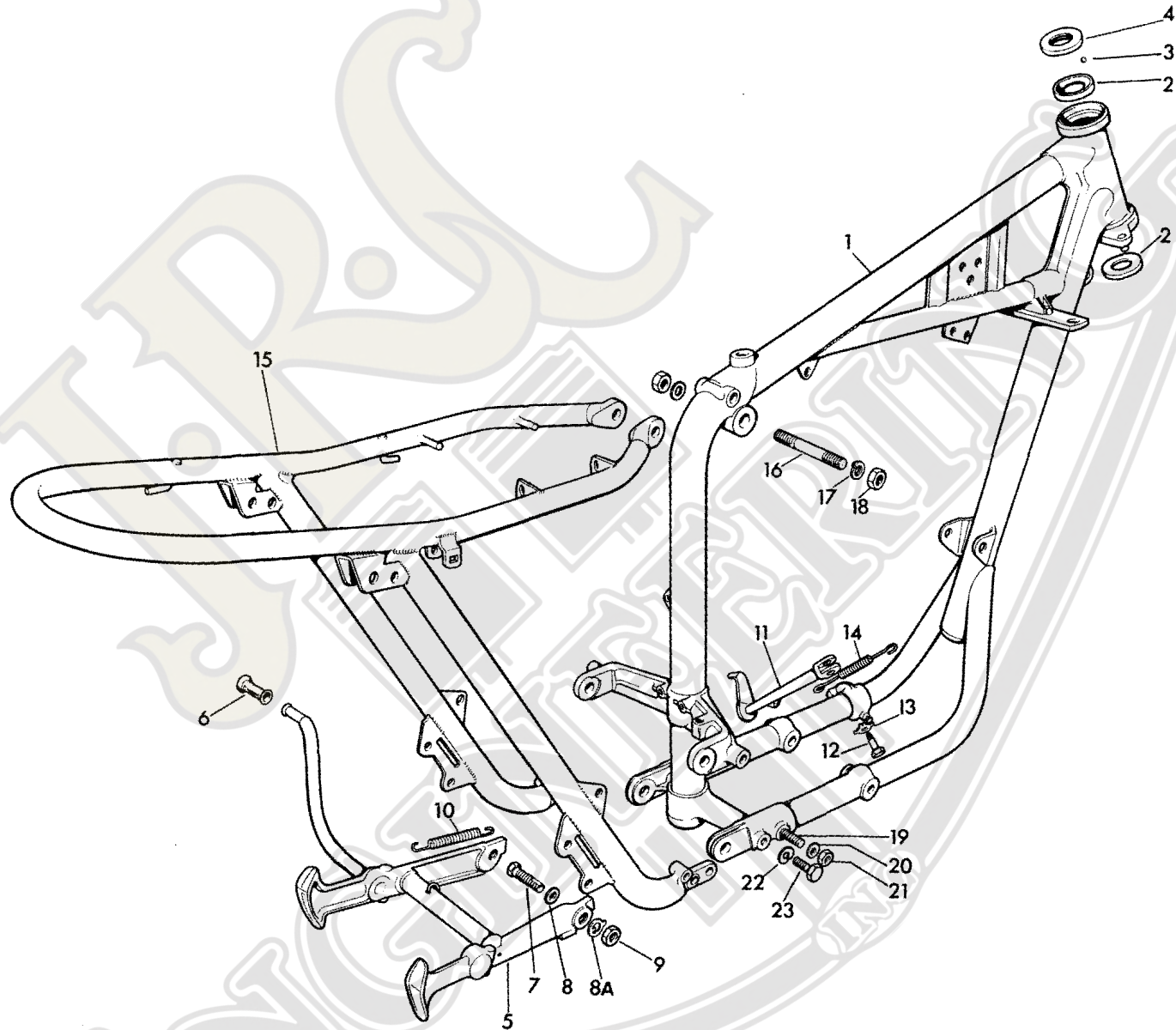
Fig. 12. FRAME
