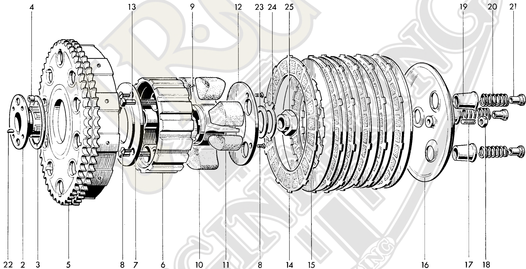
Fig. 10. CLUTCH
