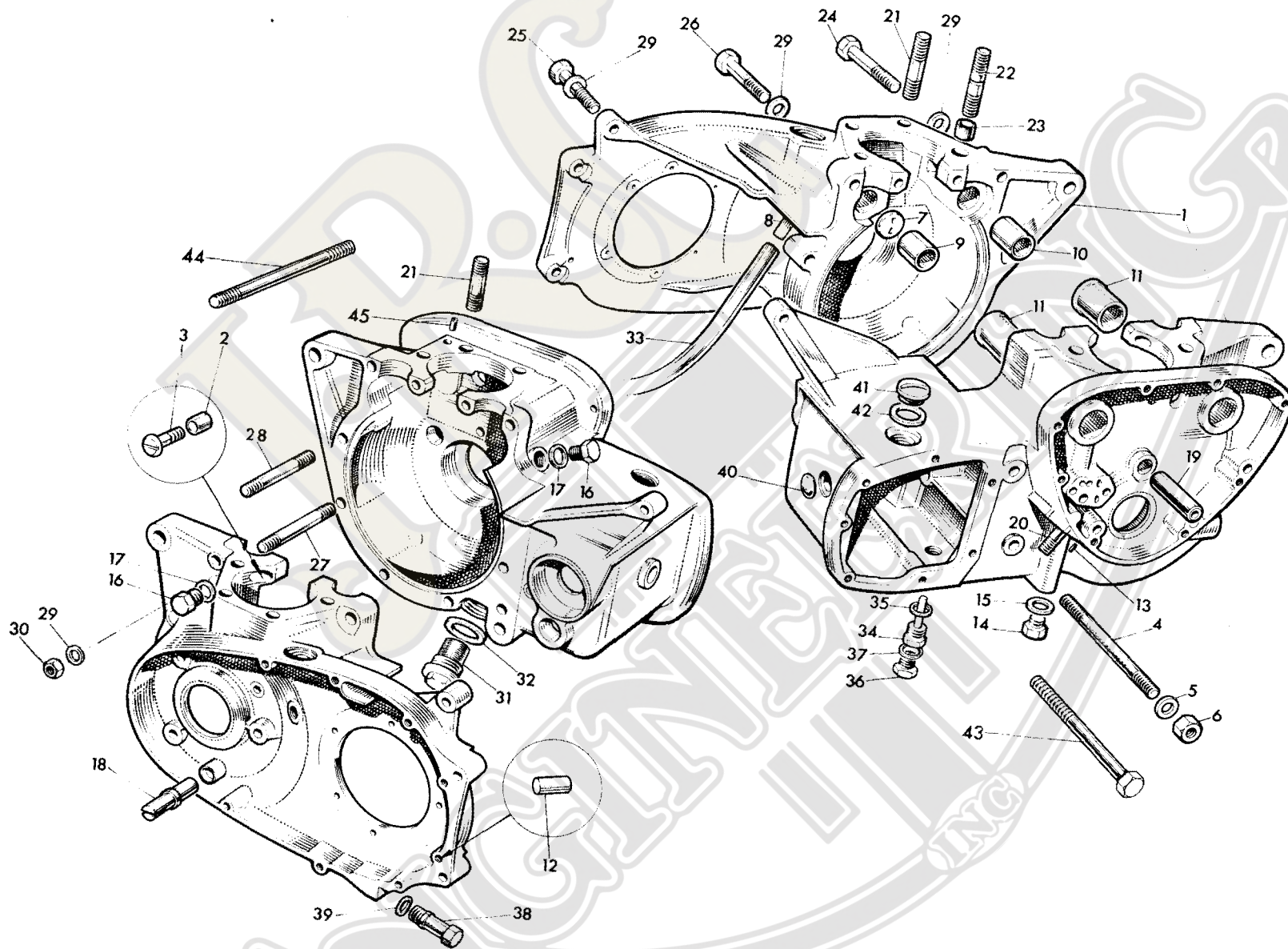
Fig. 2. CRANKCASE
