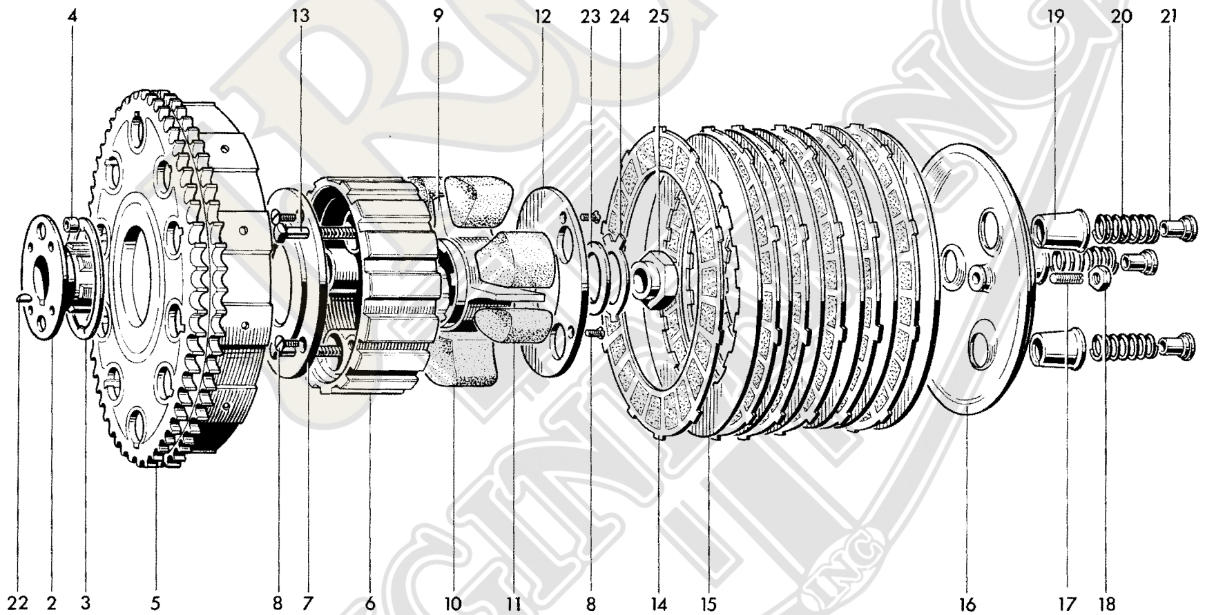
Fig. 10. CLUTCH
