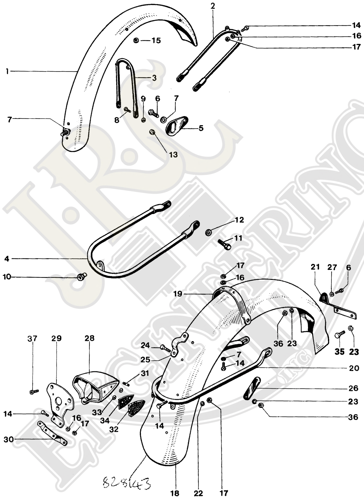
Fig. 26. FENDERS
