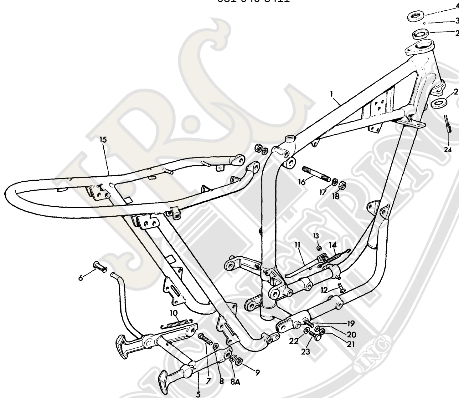
Fig. 12. FRAME
