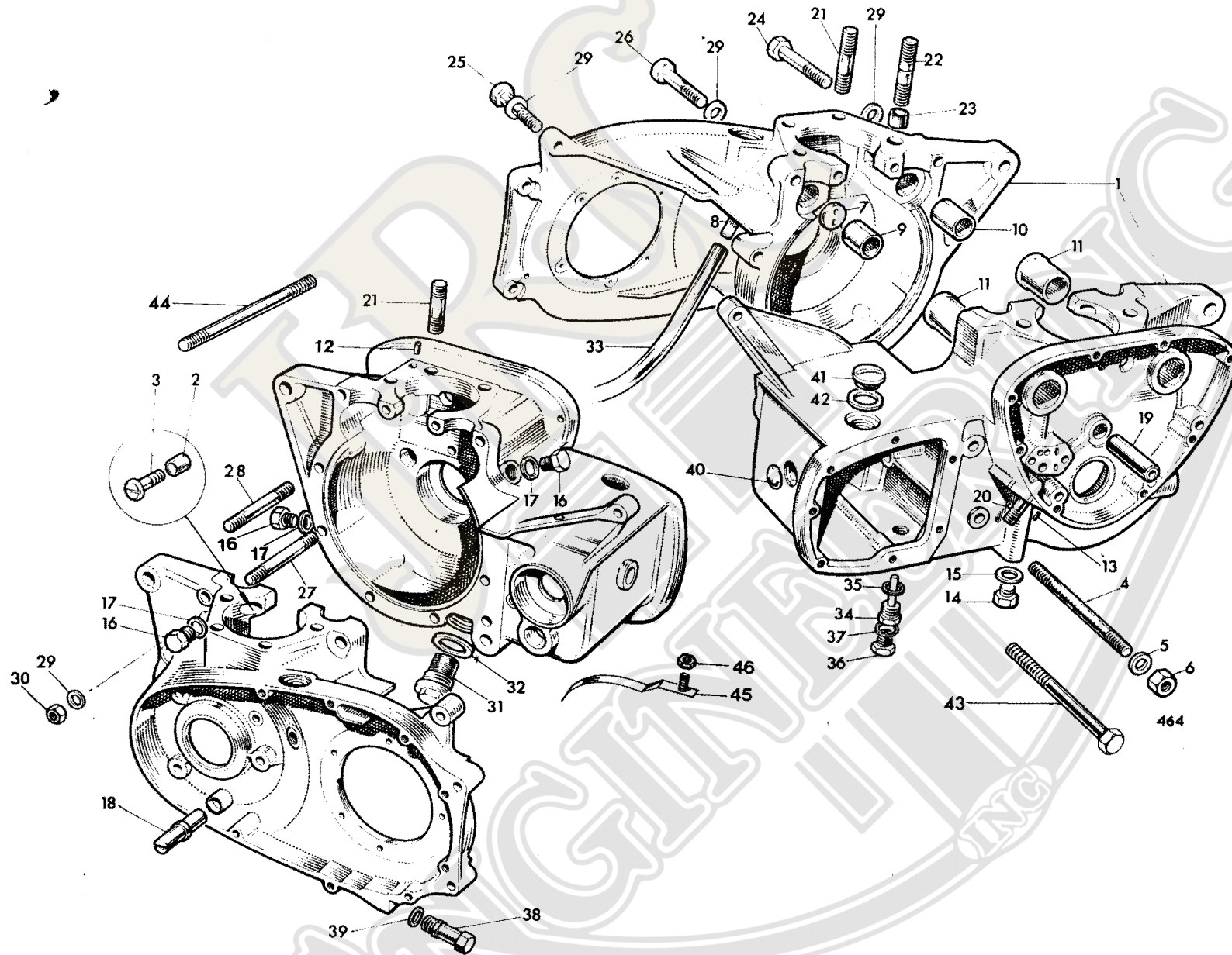
Fig. 2. CRANKCASE
