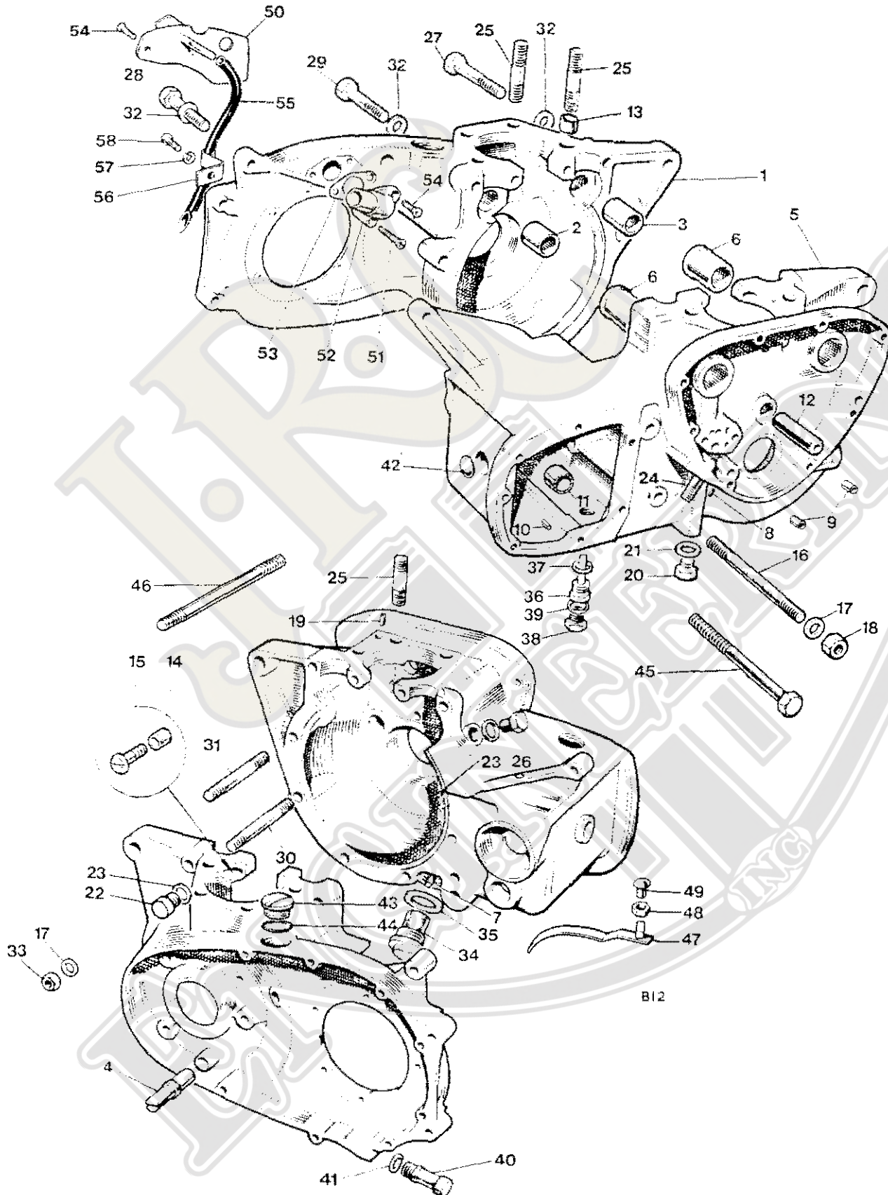
Fig. 2. CRANKCASE
