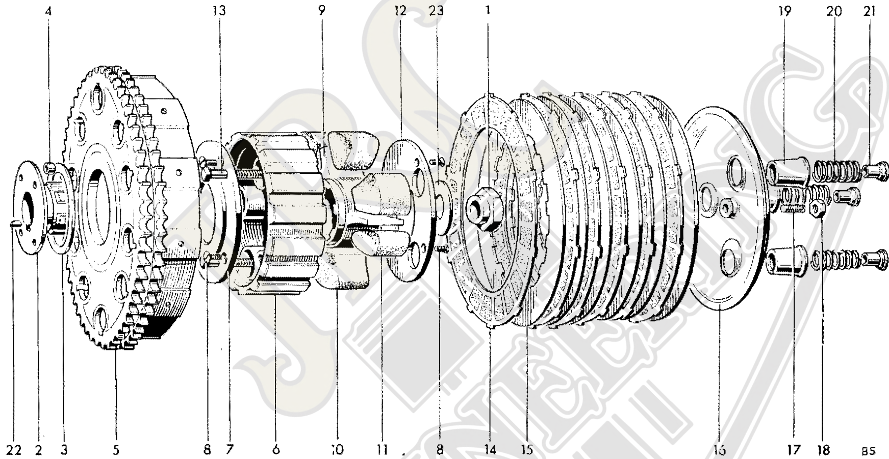
Fig. 10. CLUTCH
