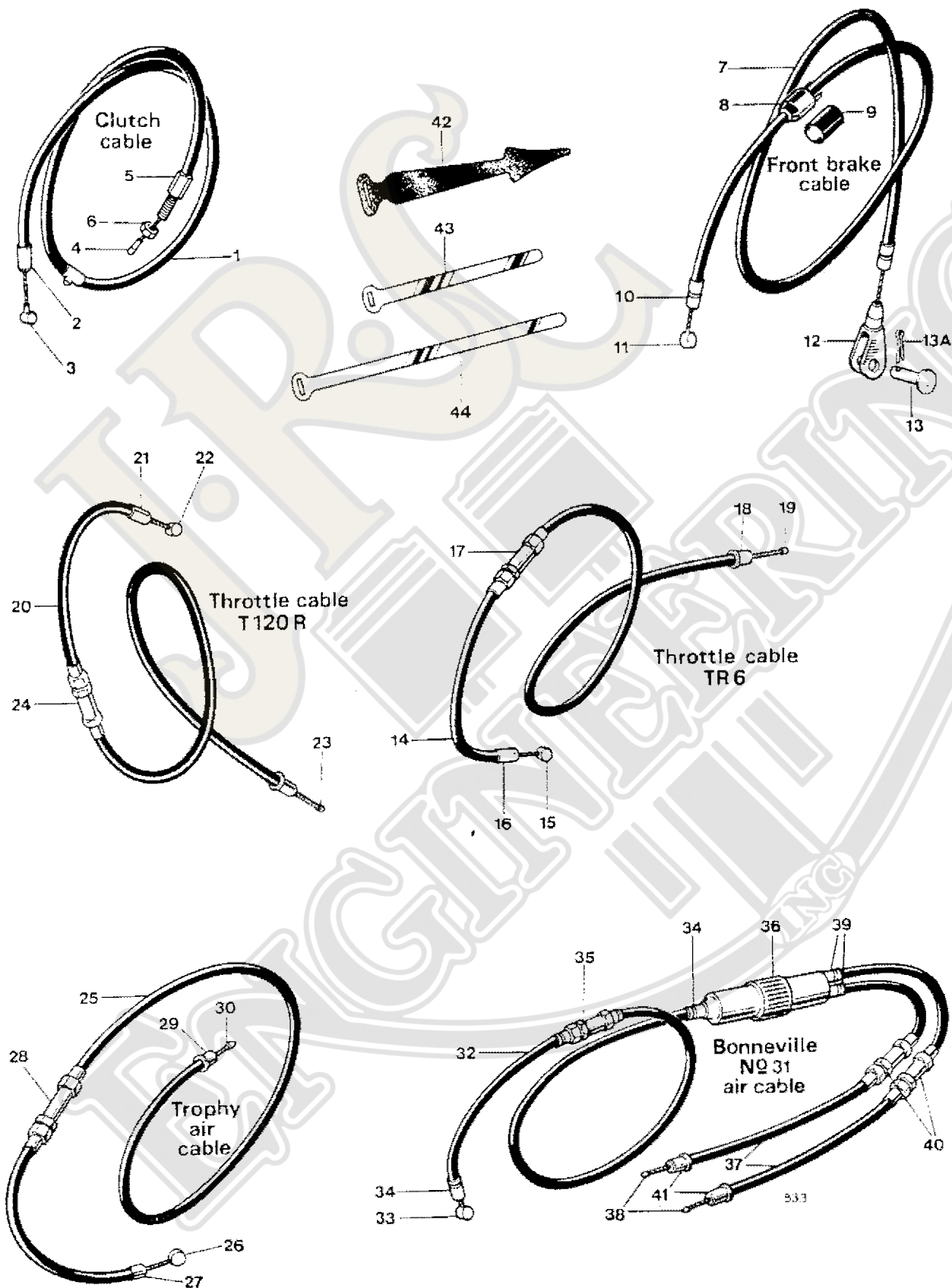
Fig. 27. CONTROL CABLES
