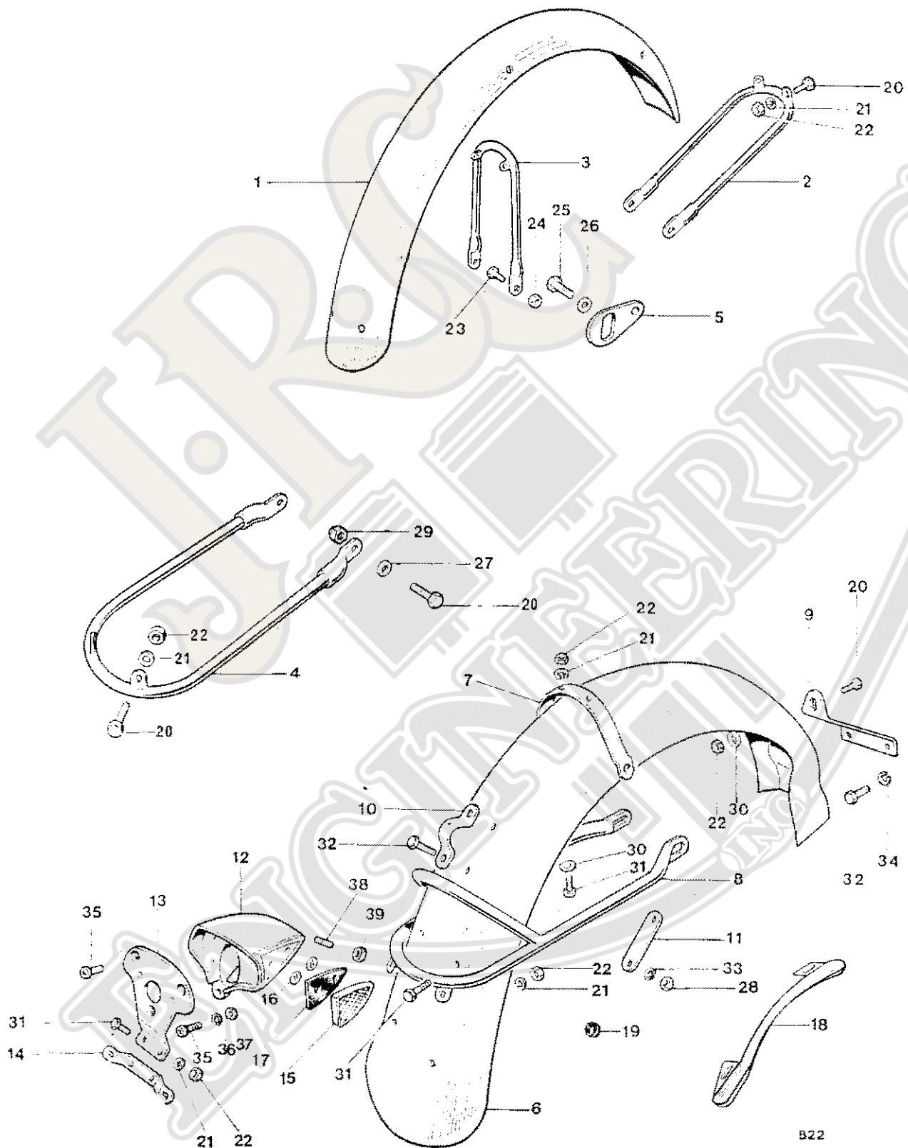
Fig. 25. FENDERS
