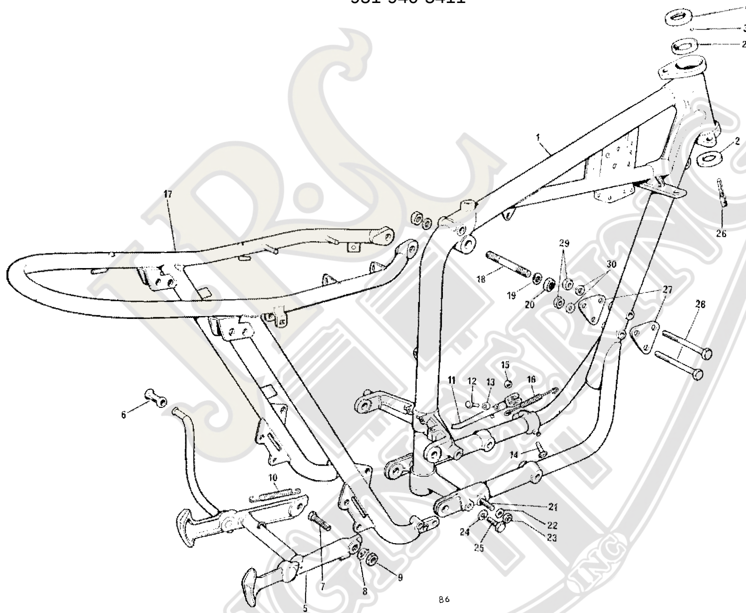
Fig. 12. FRAME
