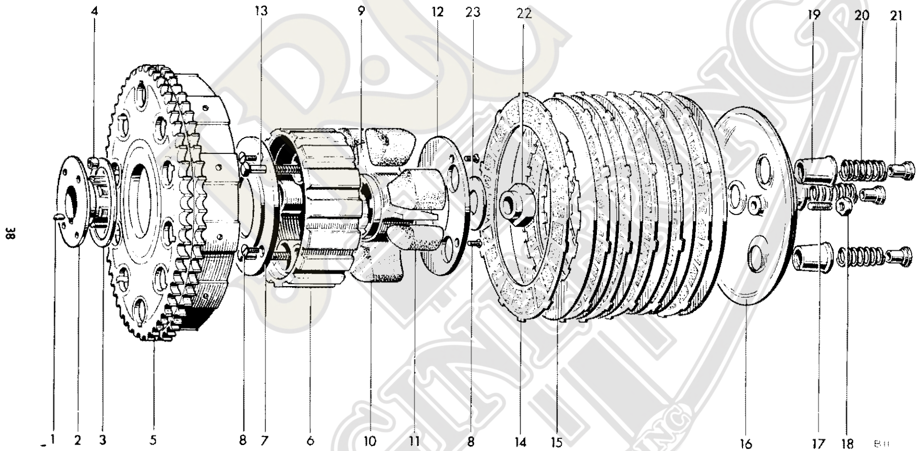
Fig. 12. CLUTCH
