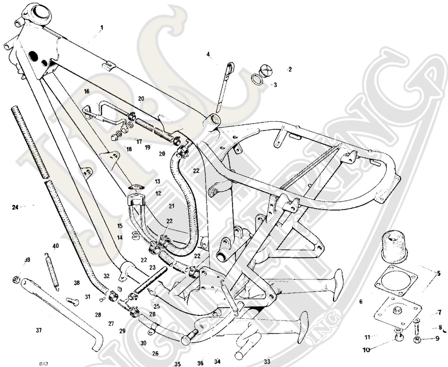
Fig. 14. FRAME
