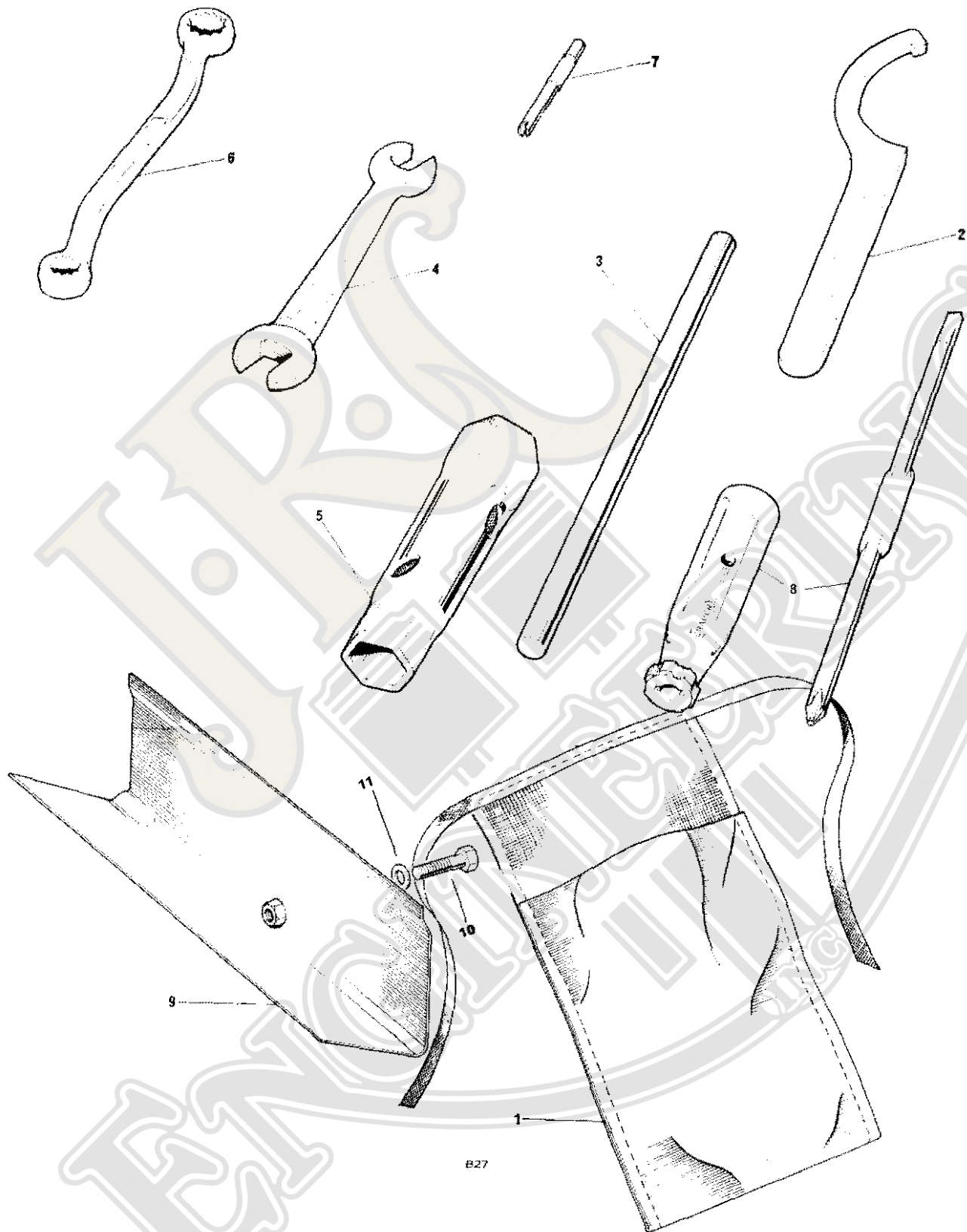
Fig. 28. TOOLKIT
