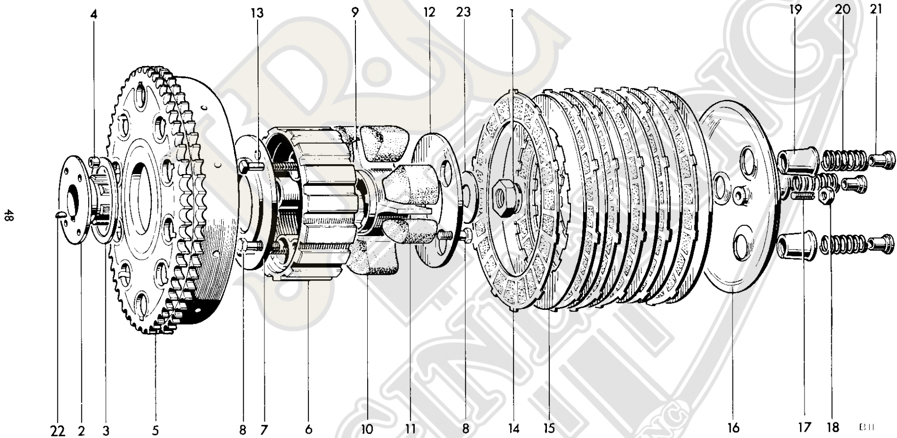
Fig. 15. CLUTCH
