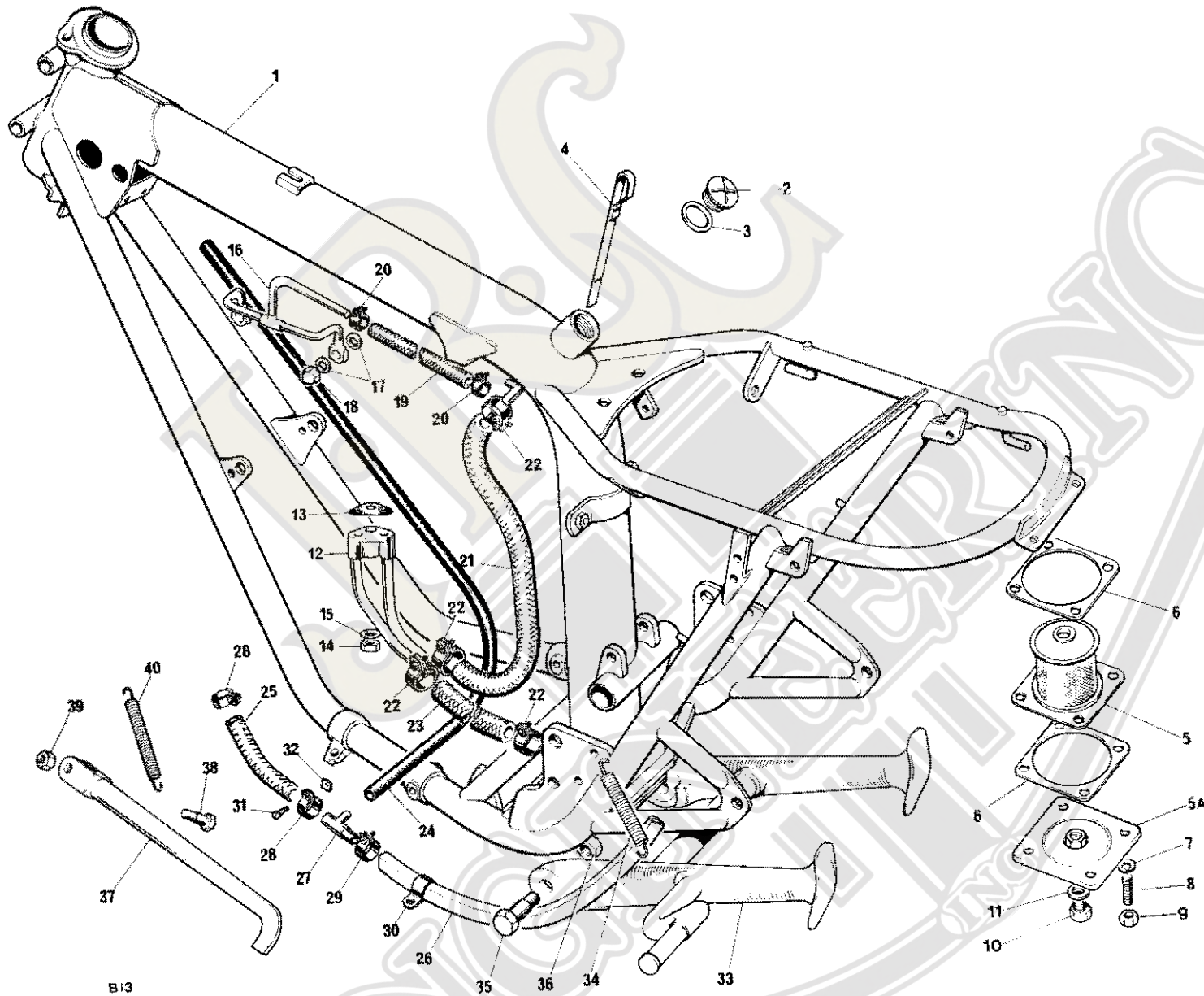
Fig. 17. FRAME
