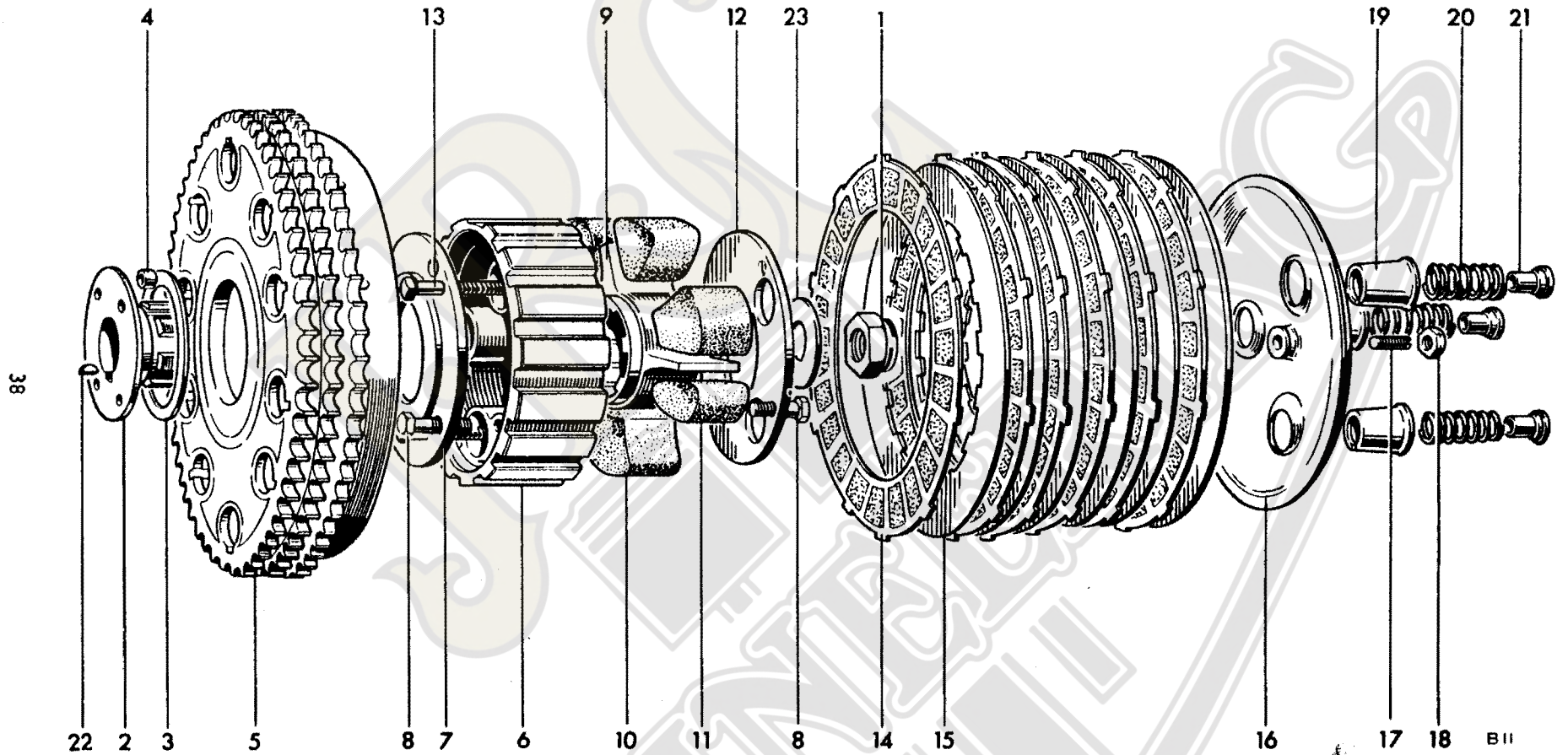
Fig. 14. CLUTCH
