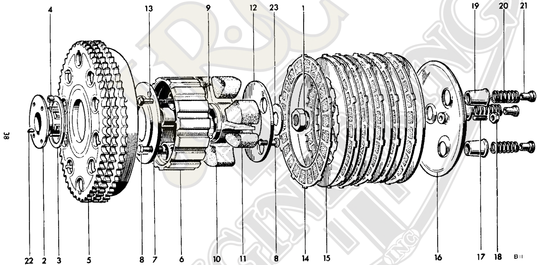
Fig. 14. CLUTCH
