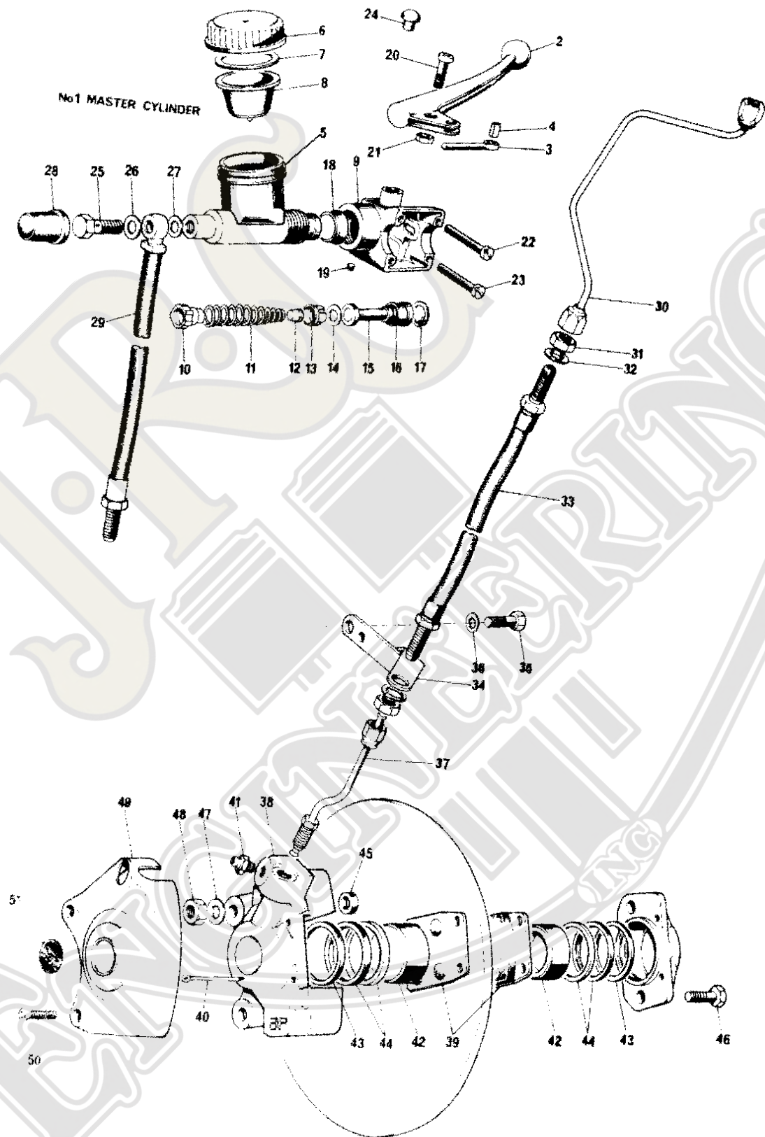
Fig. 23. FRONT BRAKE
