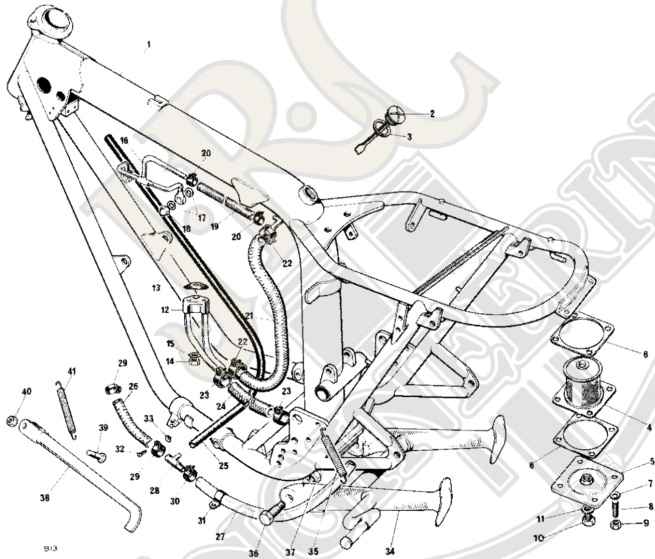
16. FRAME
