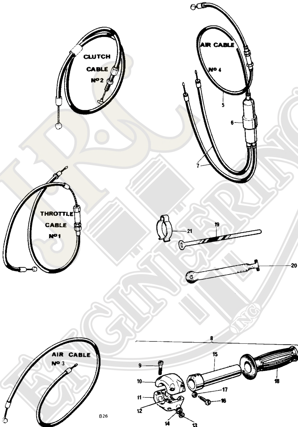
Fig. 30. CONTROL CABLES
