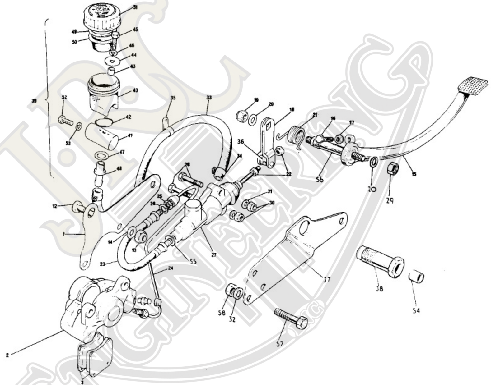
Fig. 25. REAR BRAKE
