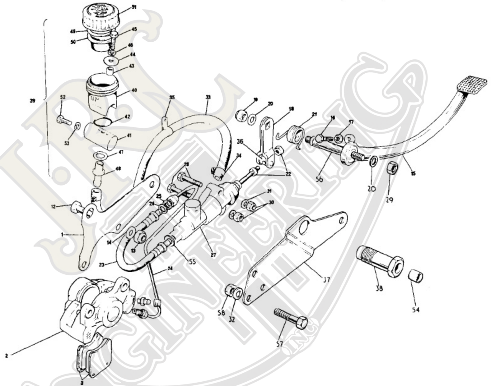
Fig. 25. REAR BRAKE
