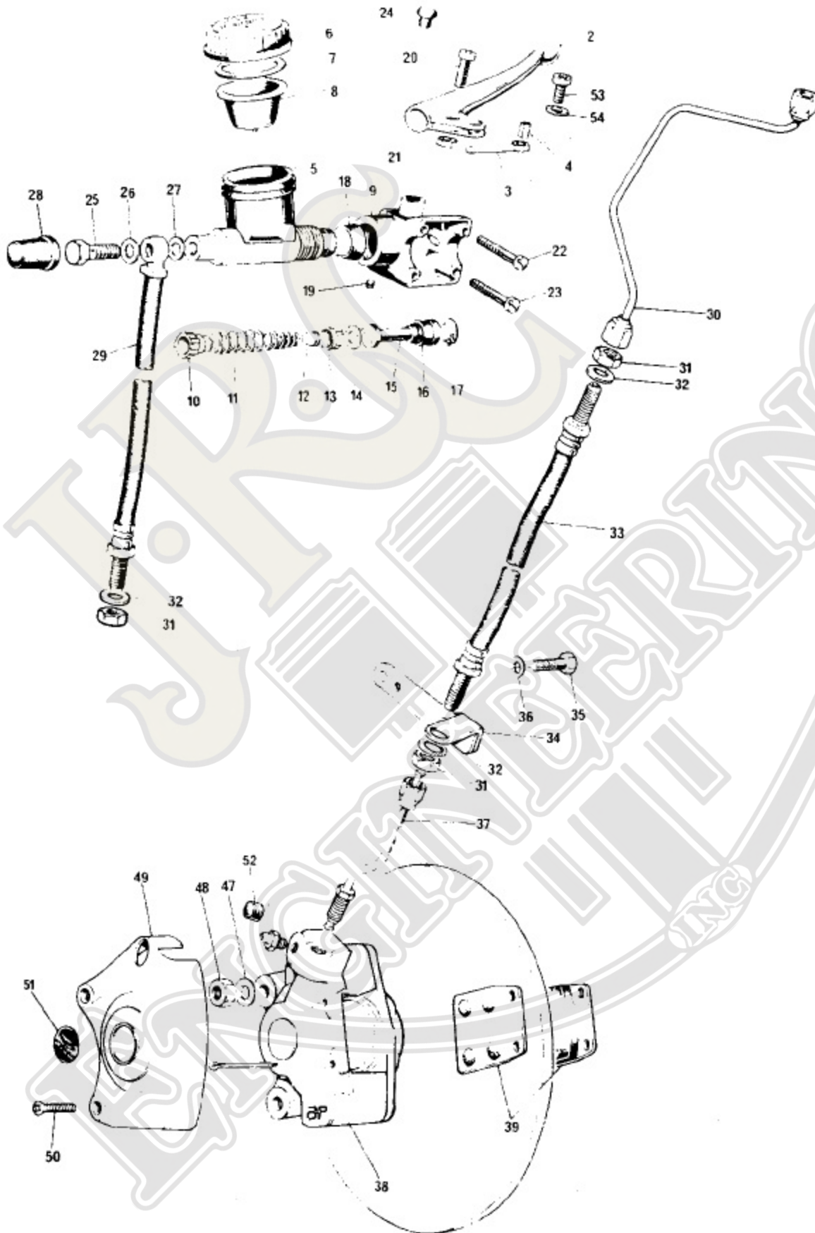
Fig. 23. FRONT BRAKE
