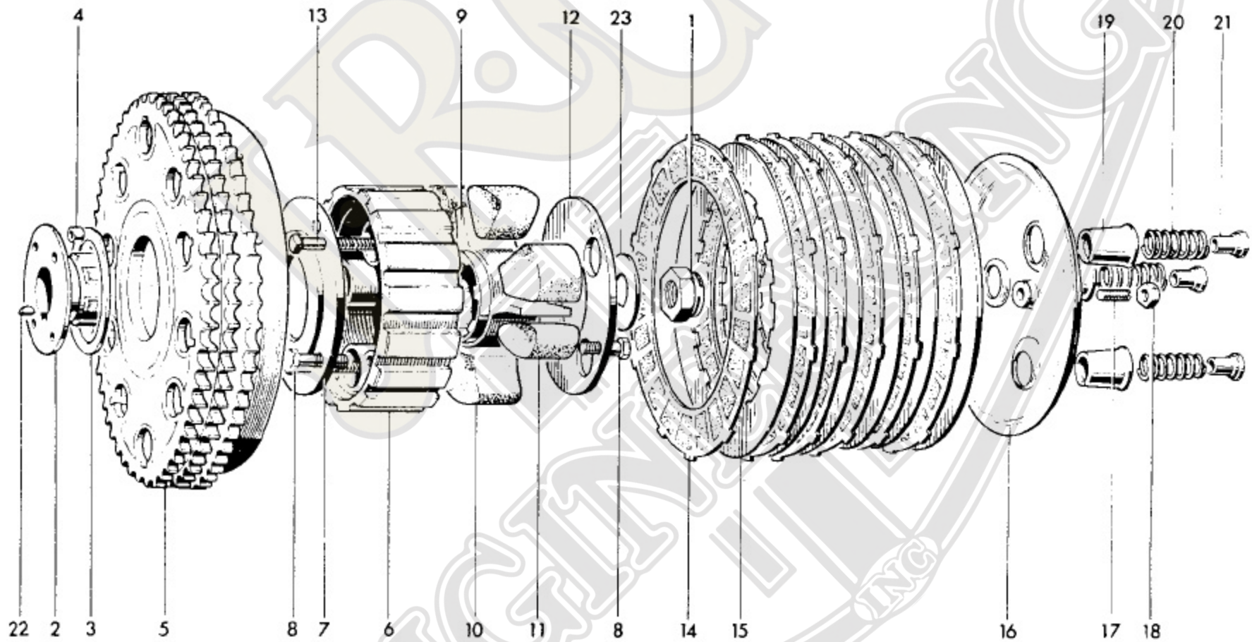
Fig. 14. CLUTCH
