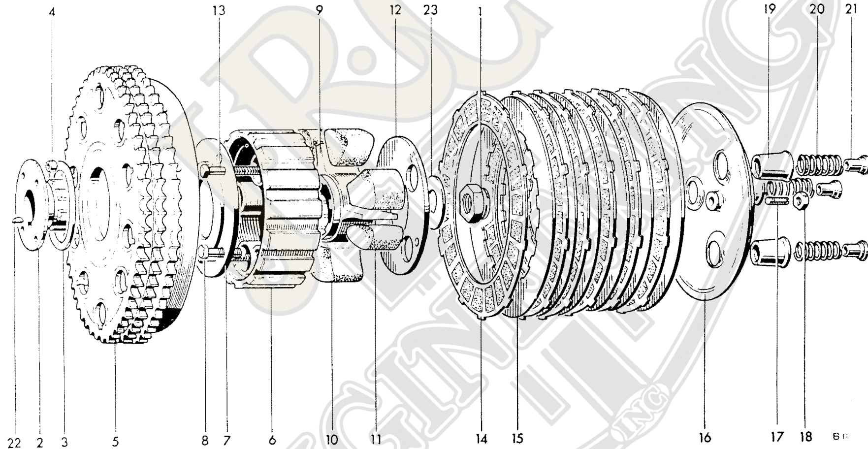
Fig. 14. CLUTCH
