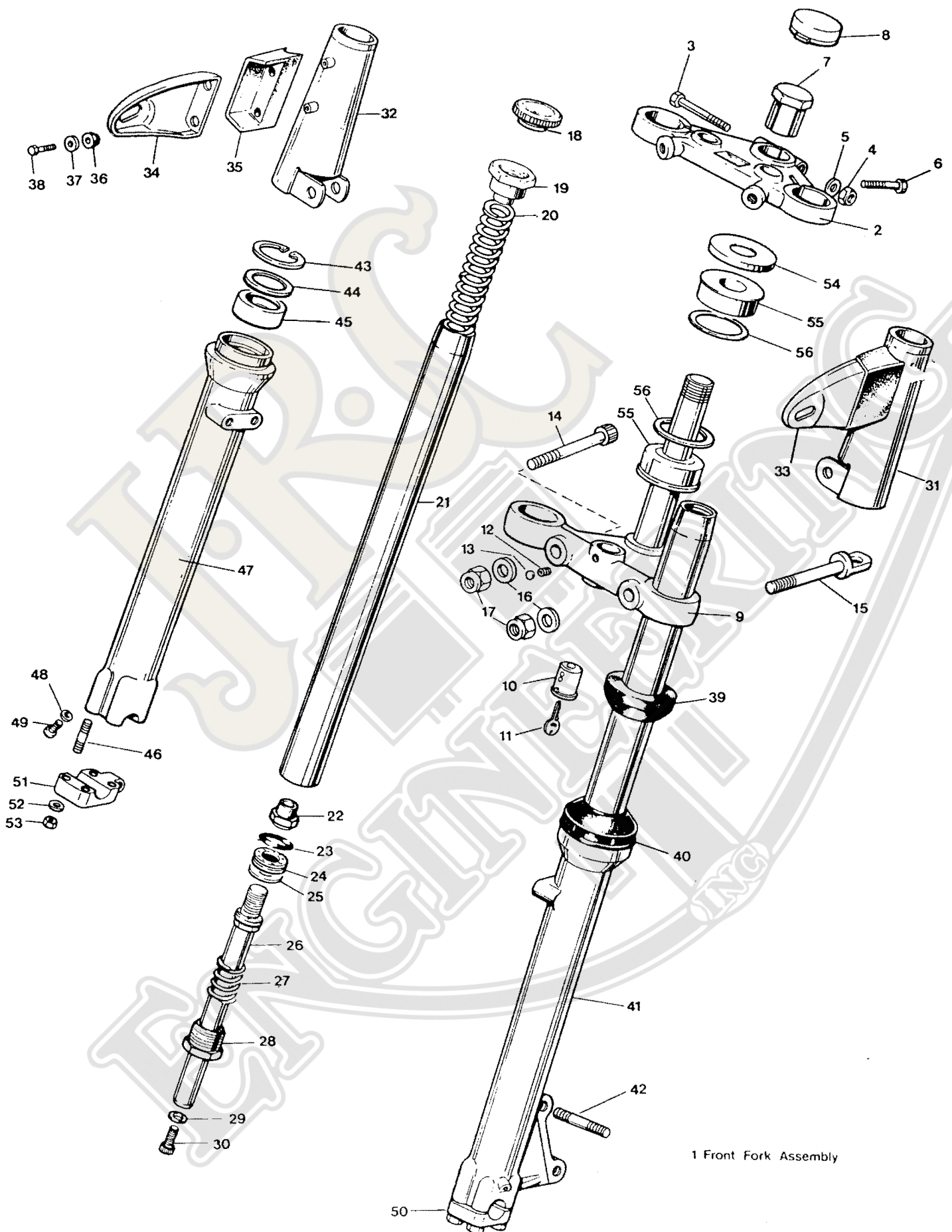
Fig. 20. TELESCOPIC FRONT FORK
