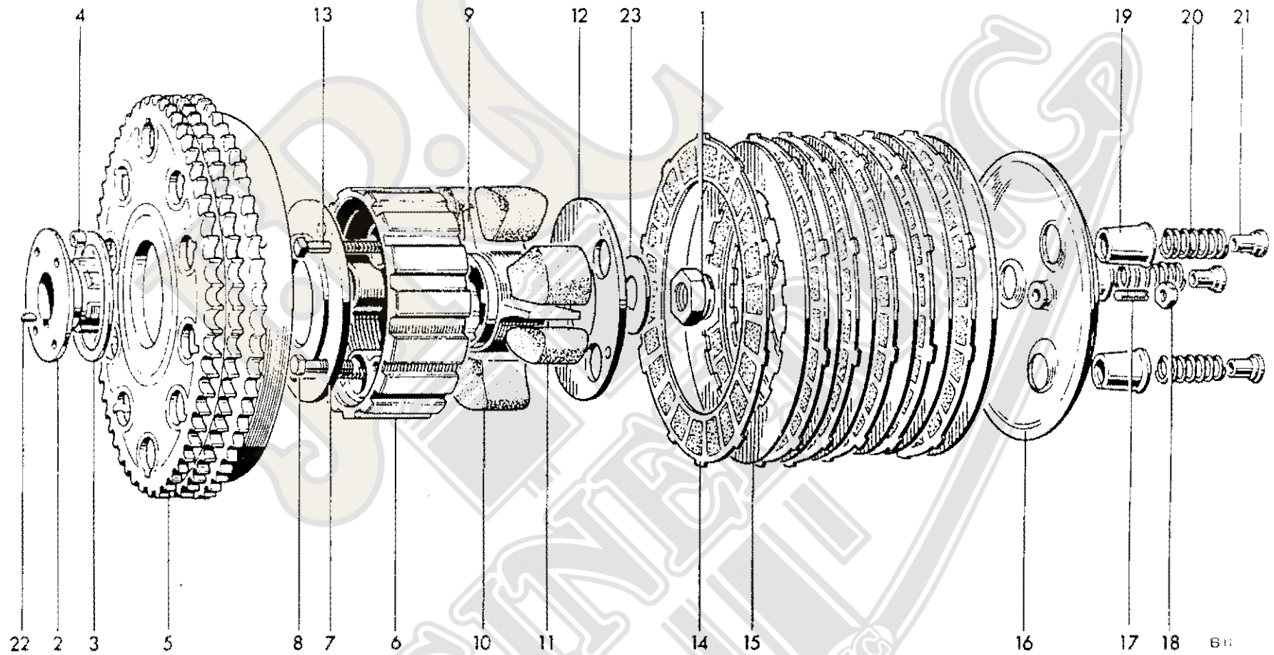
CLUTCH
