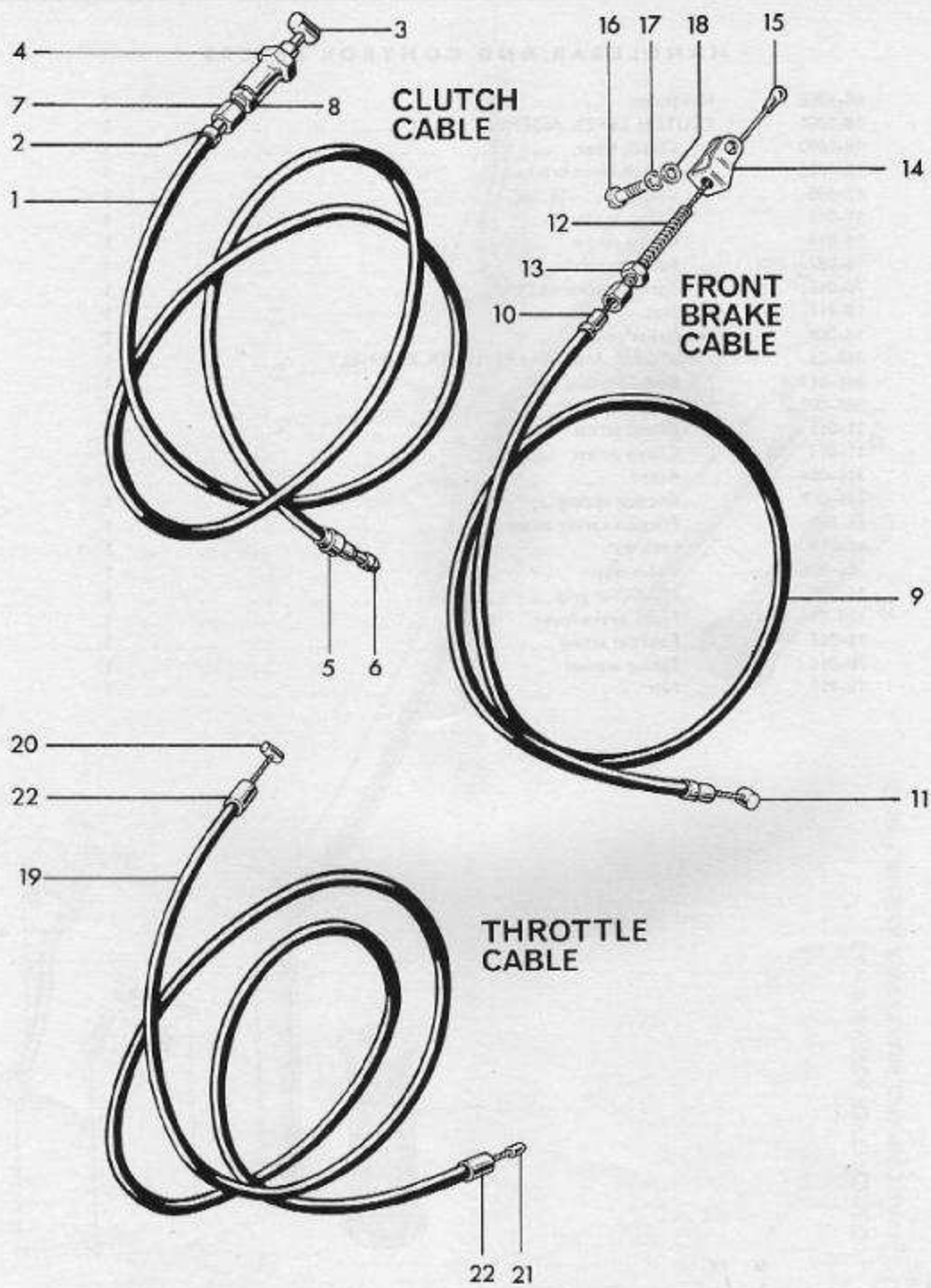
Fig. 21. CONTROL CABLES
