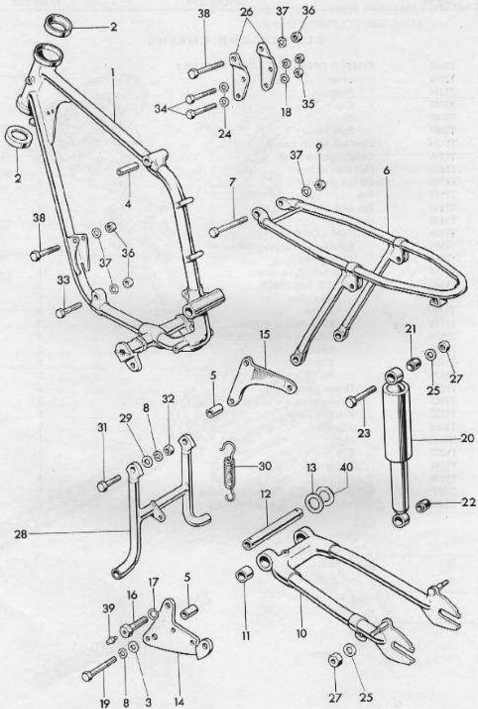
Fig. 7. FRAME COMPLETE
