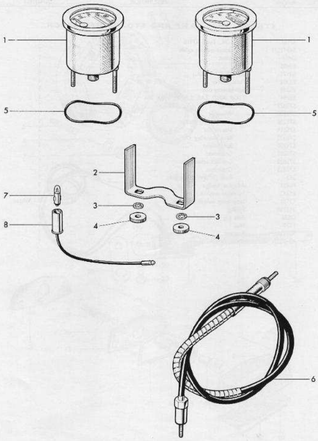
Fig. 26. SPEEDOMETER
