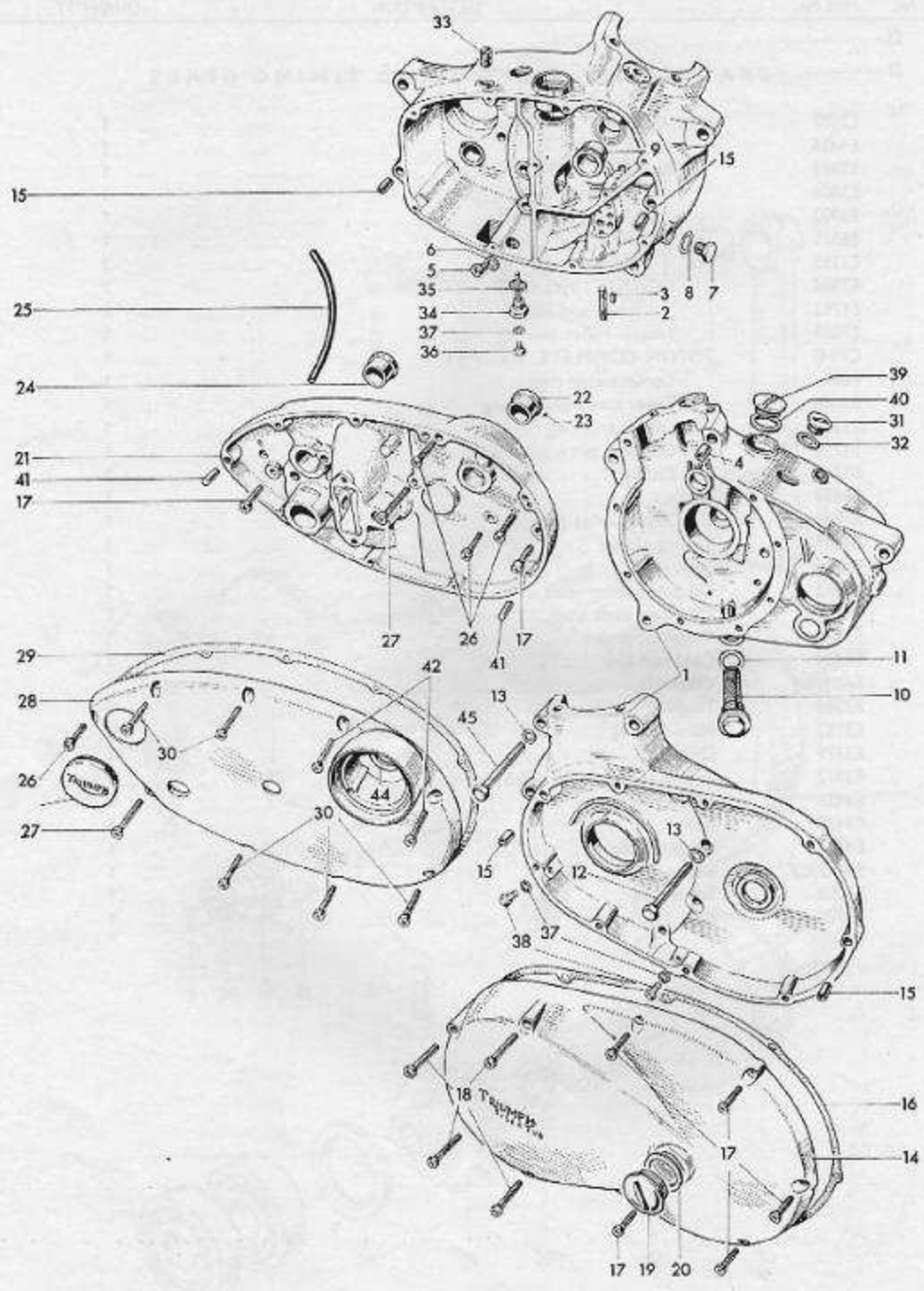
Fig. 2. CRANKCASE
