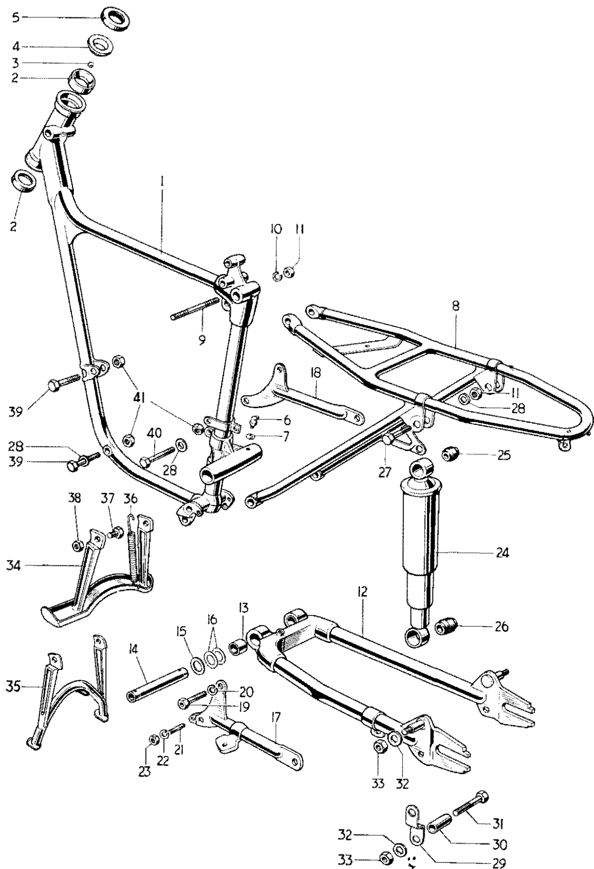
Fig. 7. FRAME COMPLETE
