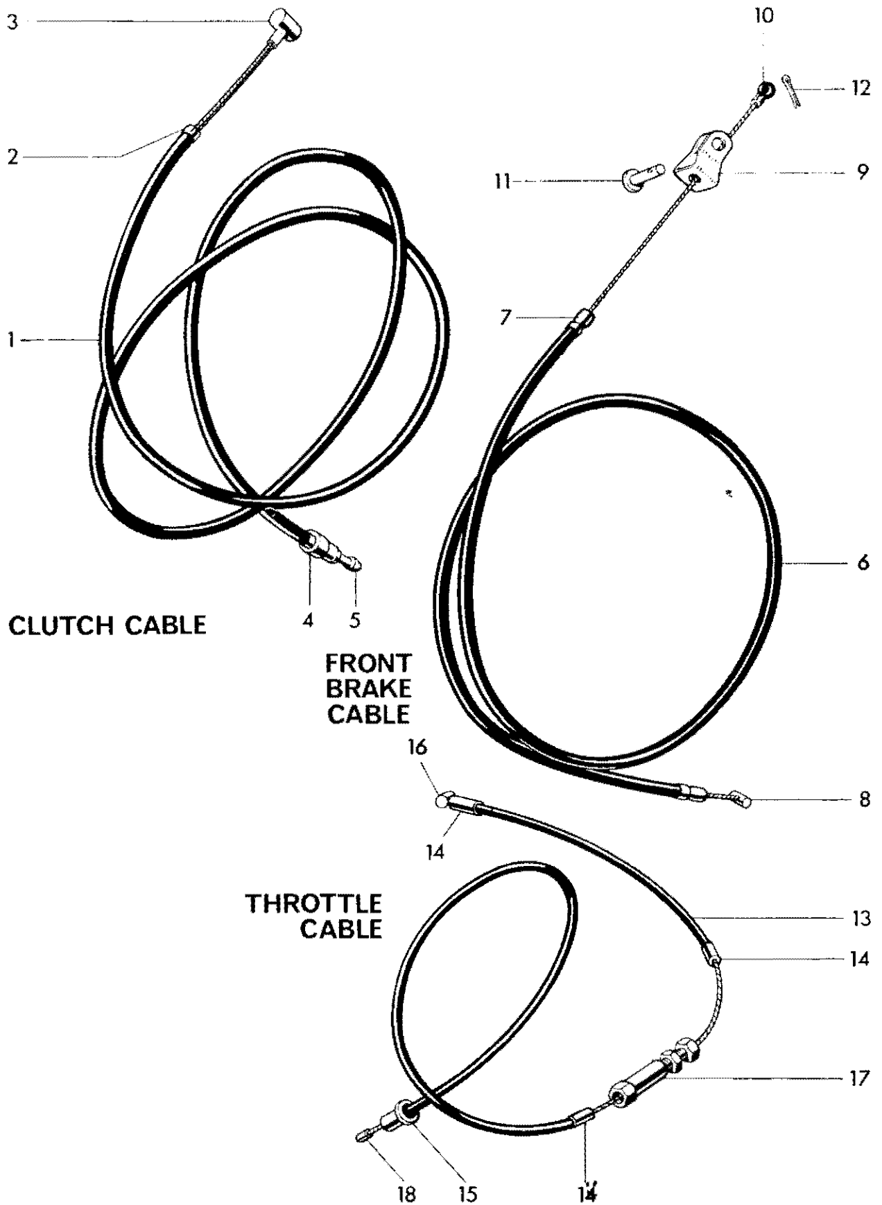
Fig. 17. CONTROL CABLES
