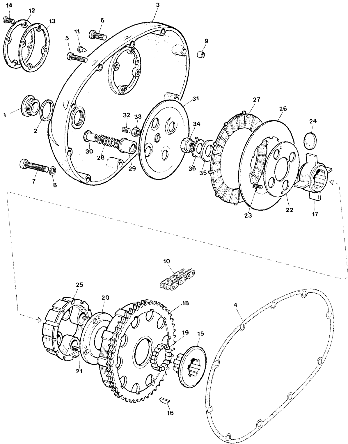
Fig. 4 CLUTCH
